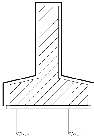
図－３ 橋梁下部
