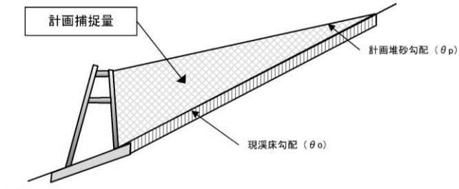
(c) 不透過型の場合
