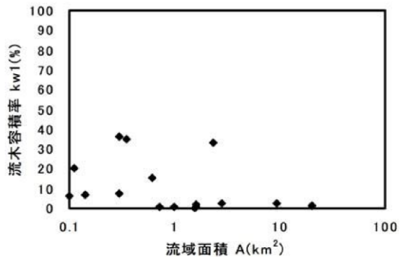
図 9-1-19 透過型砂防堰堤の流木容積率
