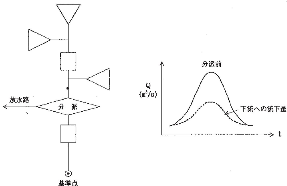
図1-10 放水路による流量配分
