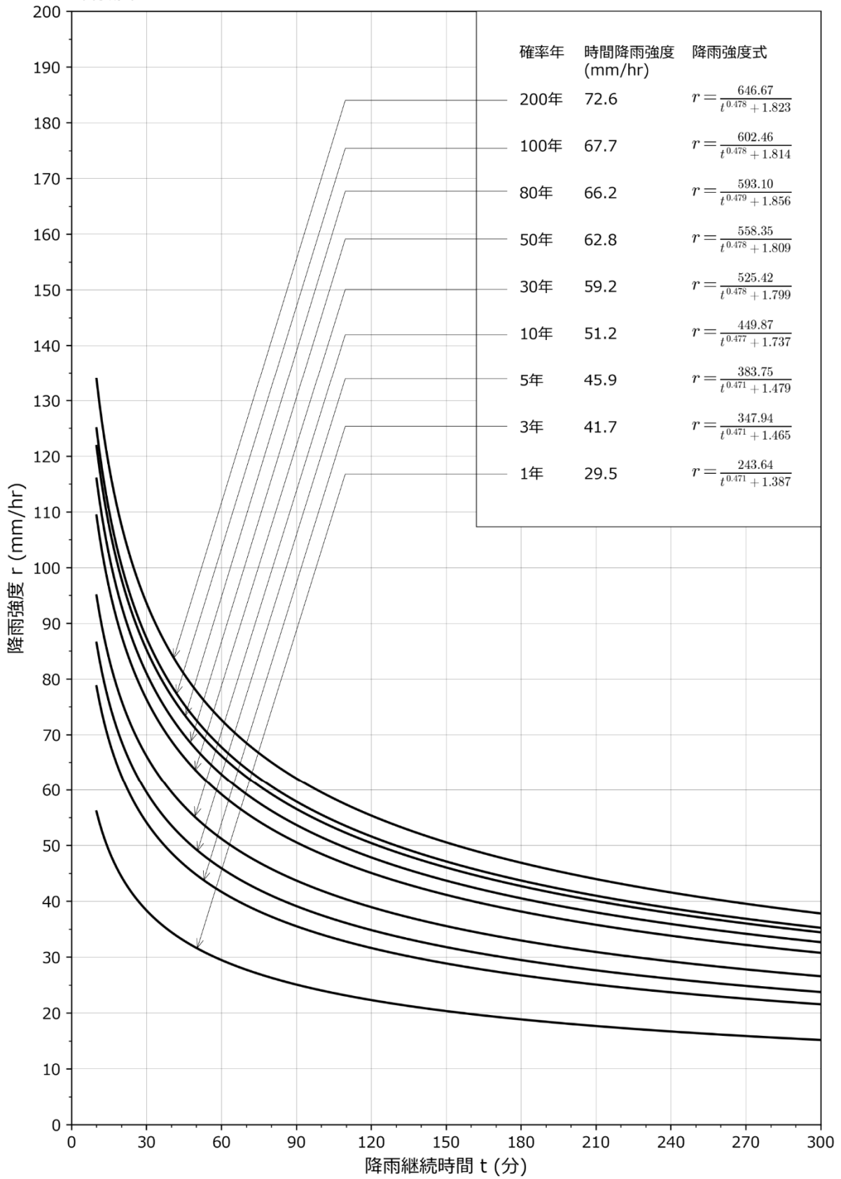
再現年別の降雨強度式と降雨強度曲線（御嶽山領域）
