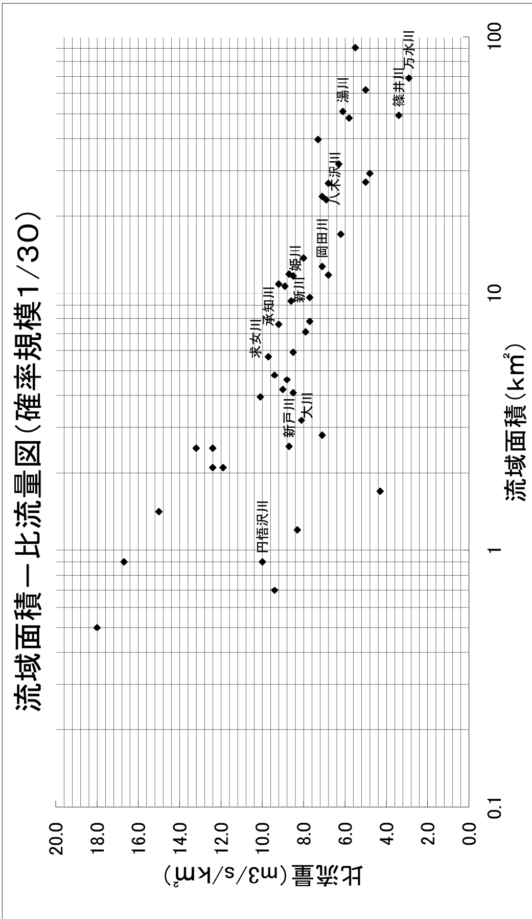
流域面積—比流量図(確率規模1/30)
