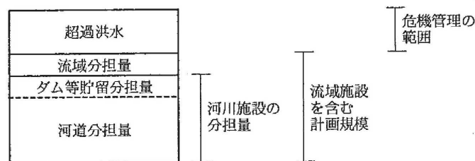
図1-6 洪水防御に対する分担と計画規模等の概念
