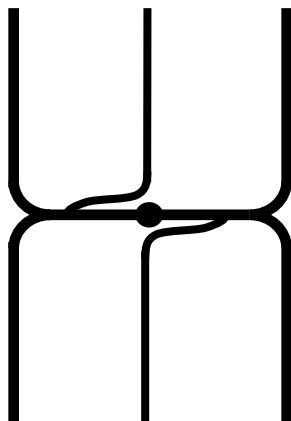
6本主枝
