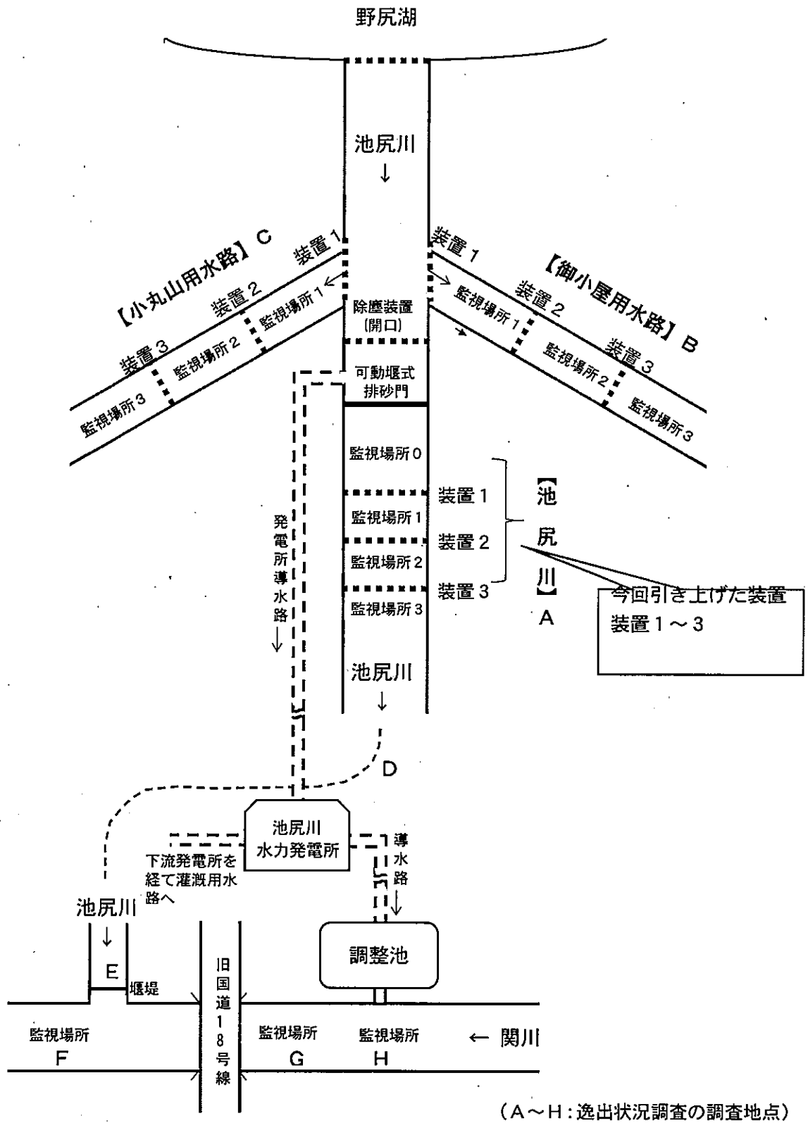
図 逸出防止施設の概要
