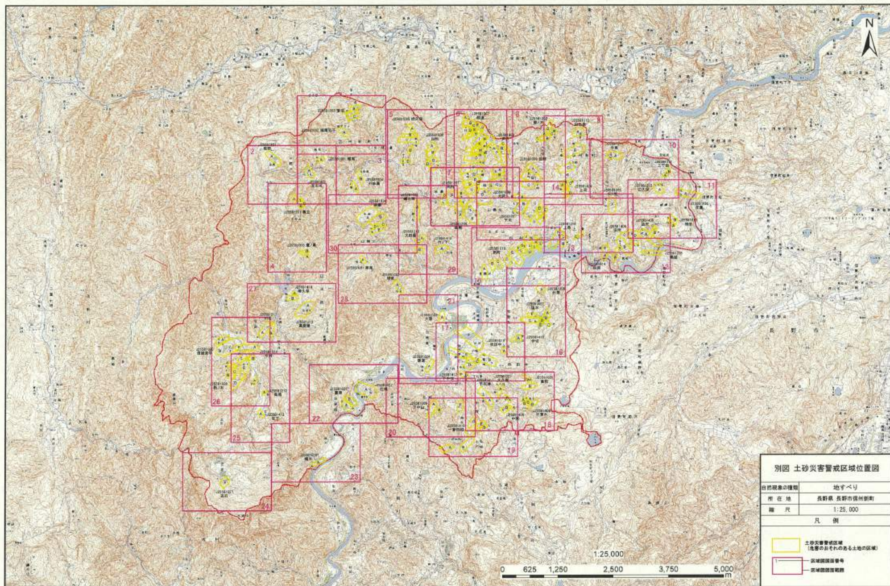
別図 土砂災害警戒区域位置図（地すべり）
