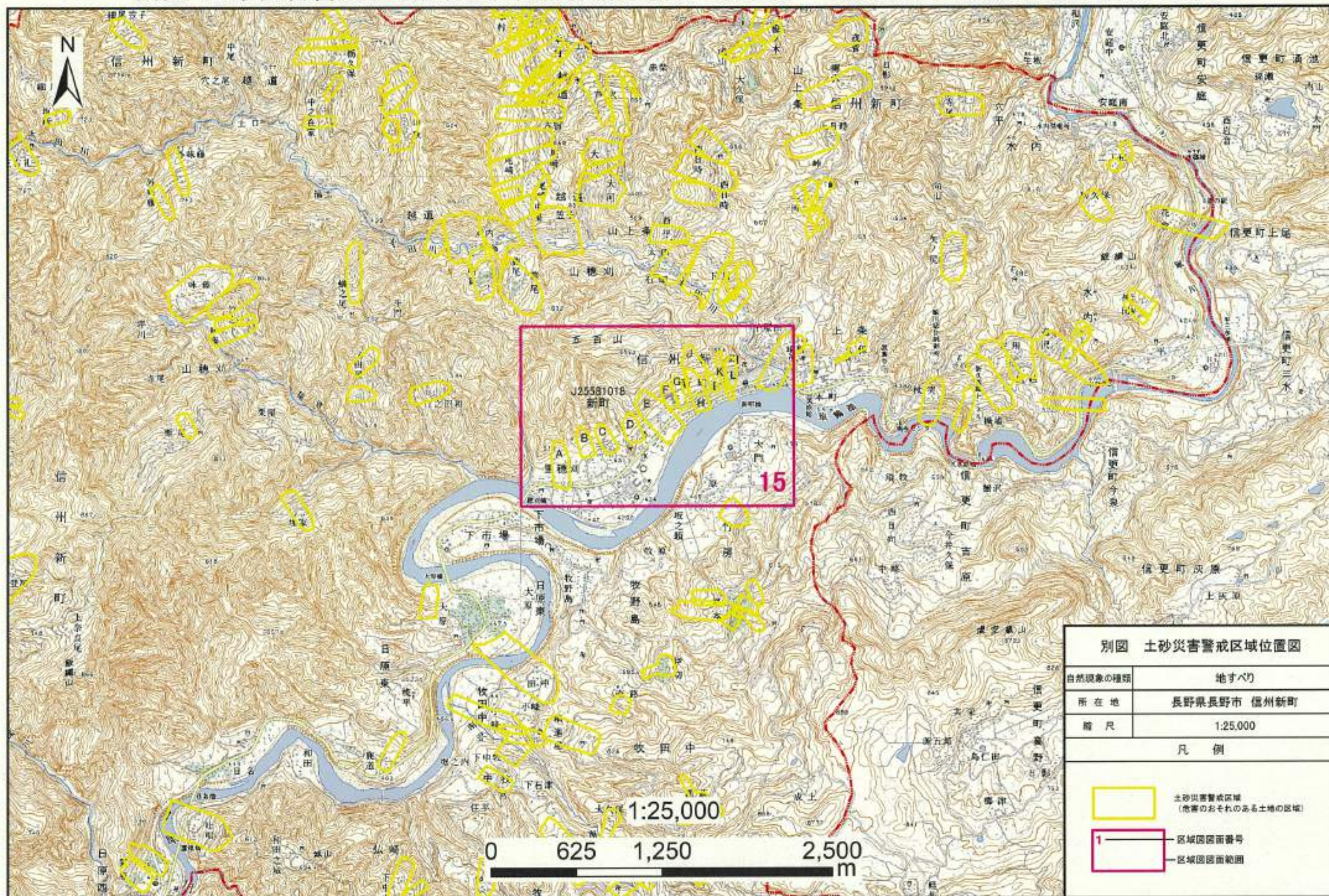
別図 土砂災害警戒区域位置図 長野市信州新町 新町第一・新町第二・里穂刈地区（地すべり）
