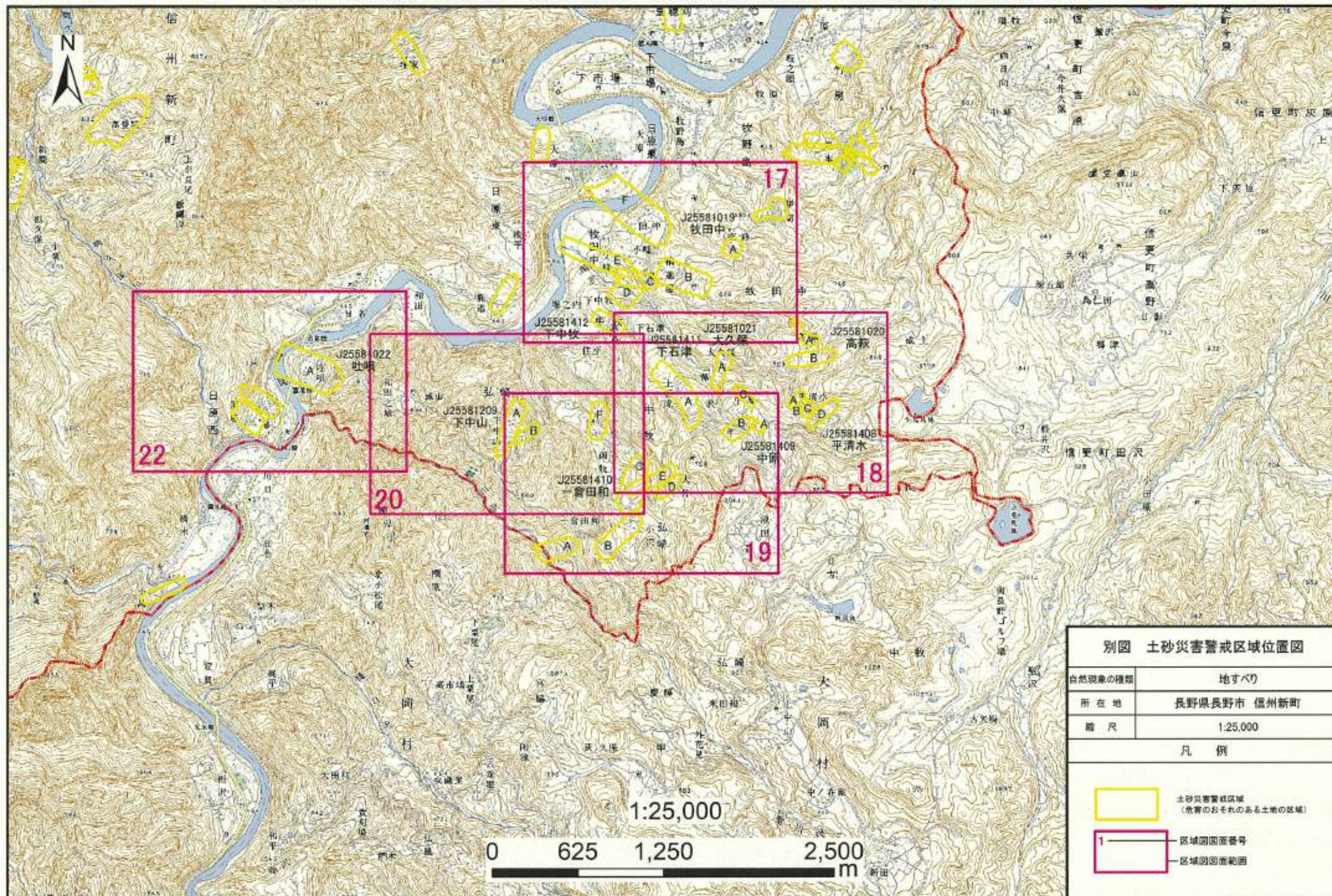
別図 土砂災害警戒区域位置図 長野市信州新町 牧南地区（地すべり）
