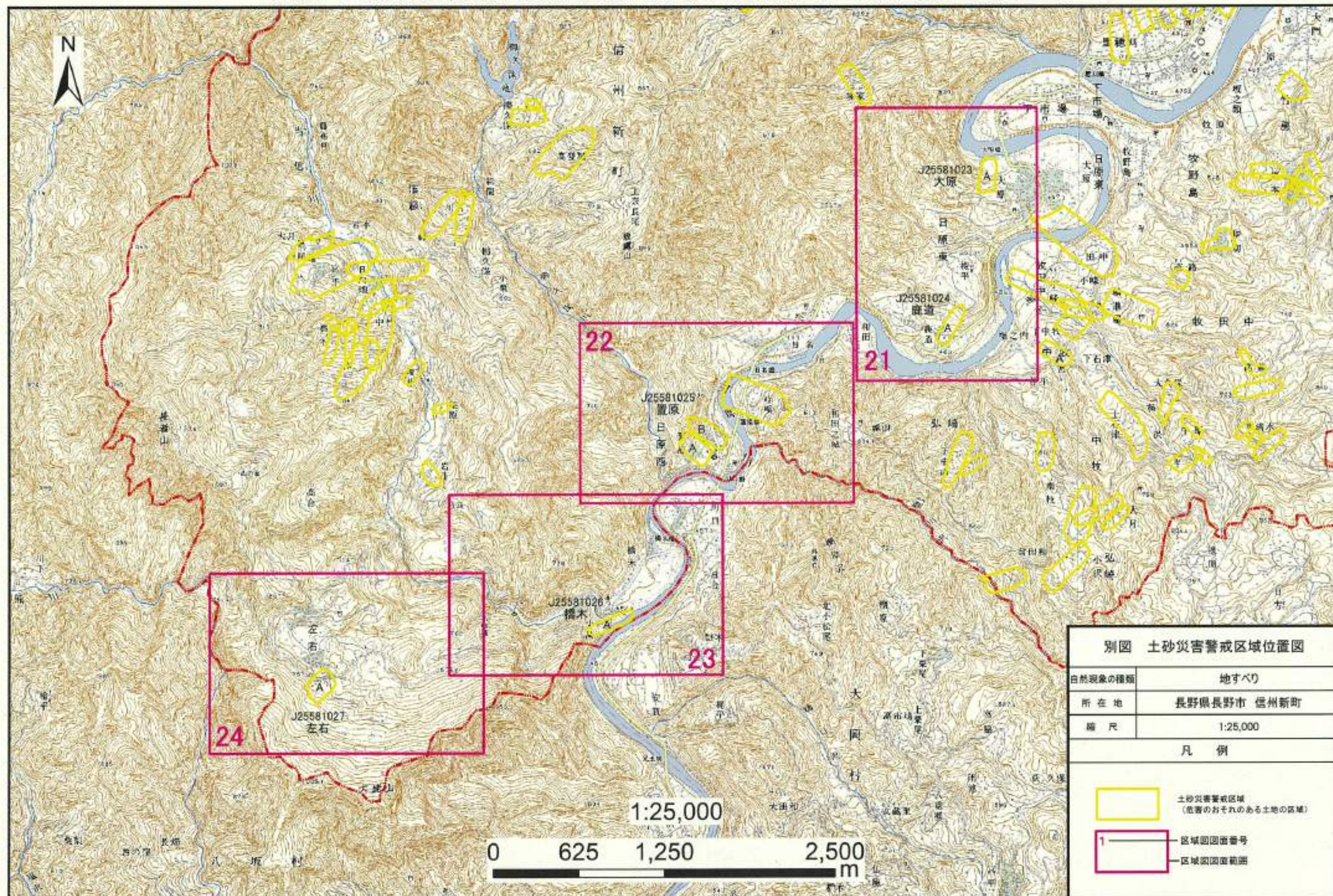
別図 土砂災害警戒区域位置図 長野市信州新町 日原地区（地すべり）
