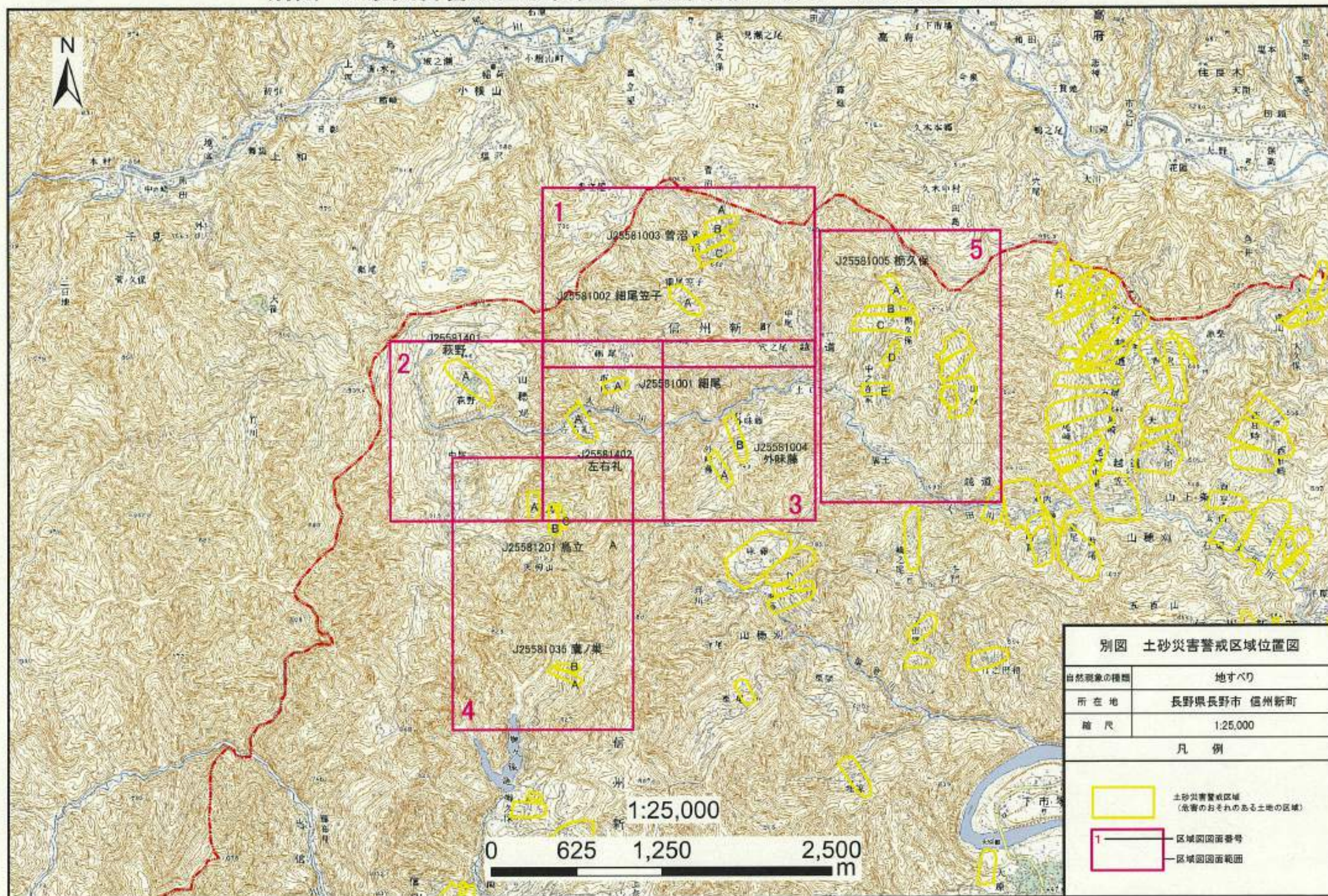
別図 土砂災害警戒区域位置図 長野市信州新町 西部地区（地すべり）
