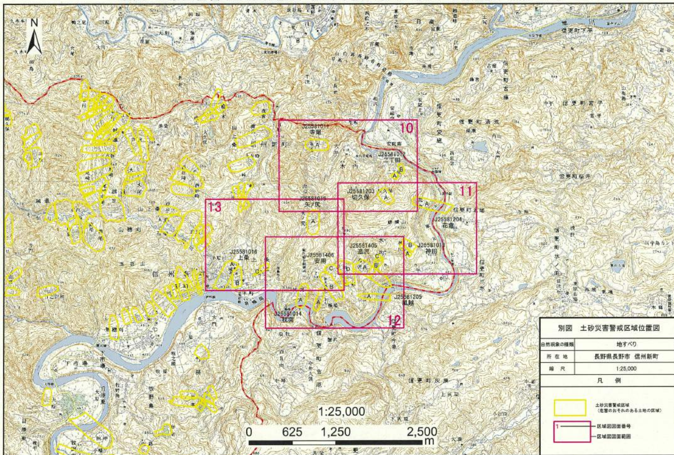
別図 土砂災害警戒区域位置図 長野市信州新町 水内・上条地区（地すべり）
