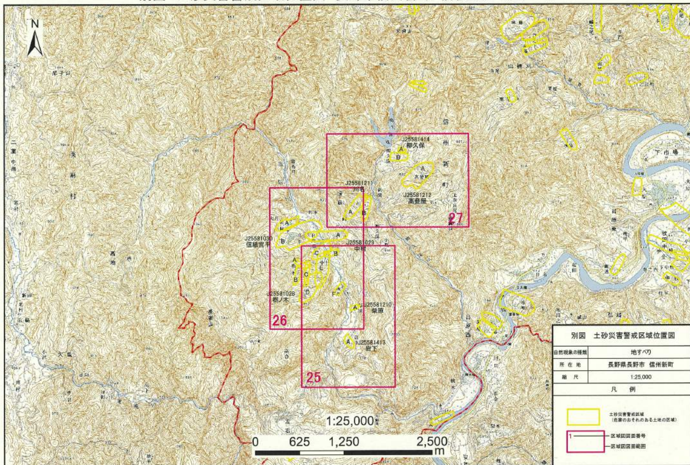
別図 土砂災害警戒区域位置図 長野市信州新町 信級地区（地すべり）
