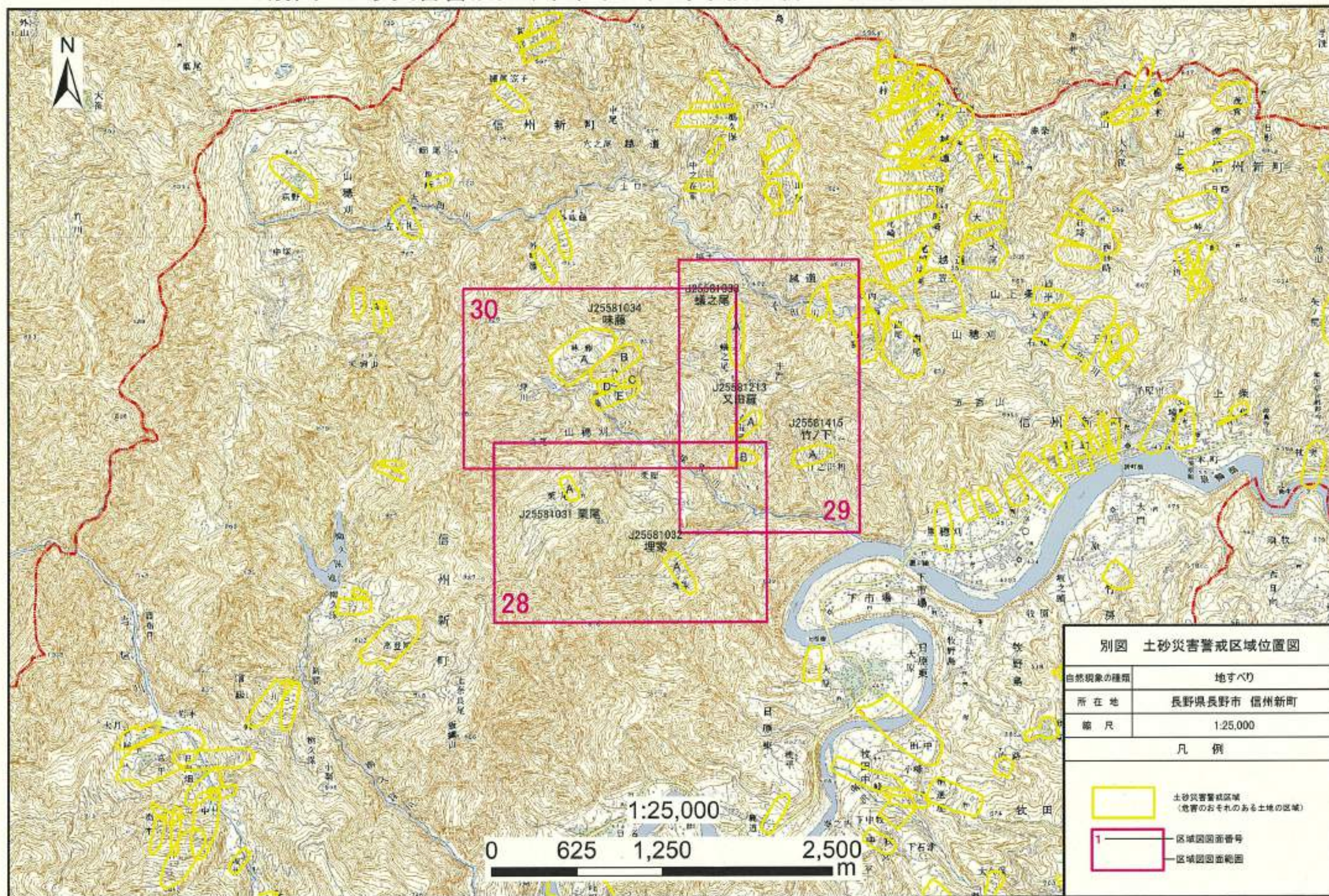
別図 土砂災害警戒区域位置図 長野市信州新町 南部地区（地すべり）
