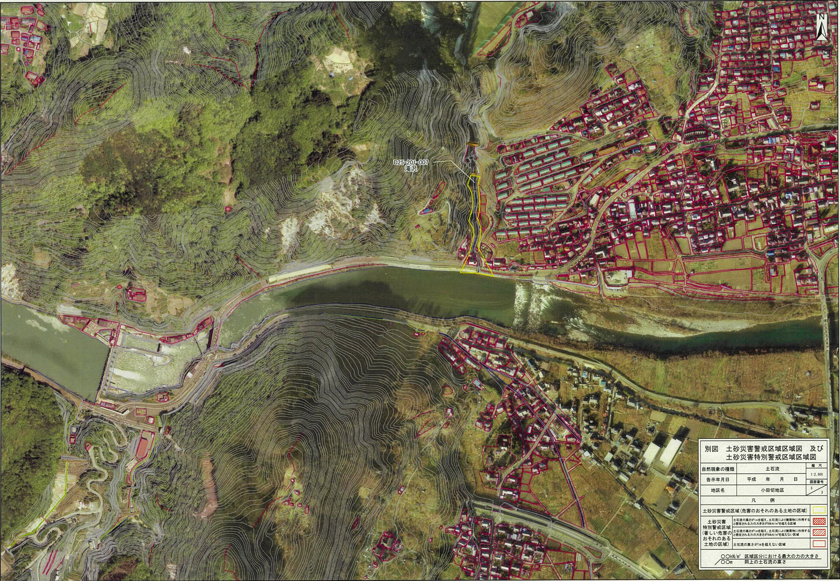
土砂災害警戒区域区域図及び土砂災害特別警戒区域区域図(土石流) 長野市小田切地区
