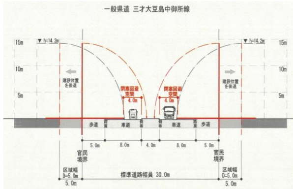
【(一) 三才大豆島中御所線 (標準断面図)】
