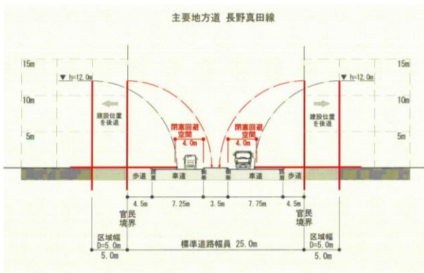
【(主) 長野真田線 (標準断面図)】
