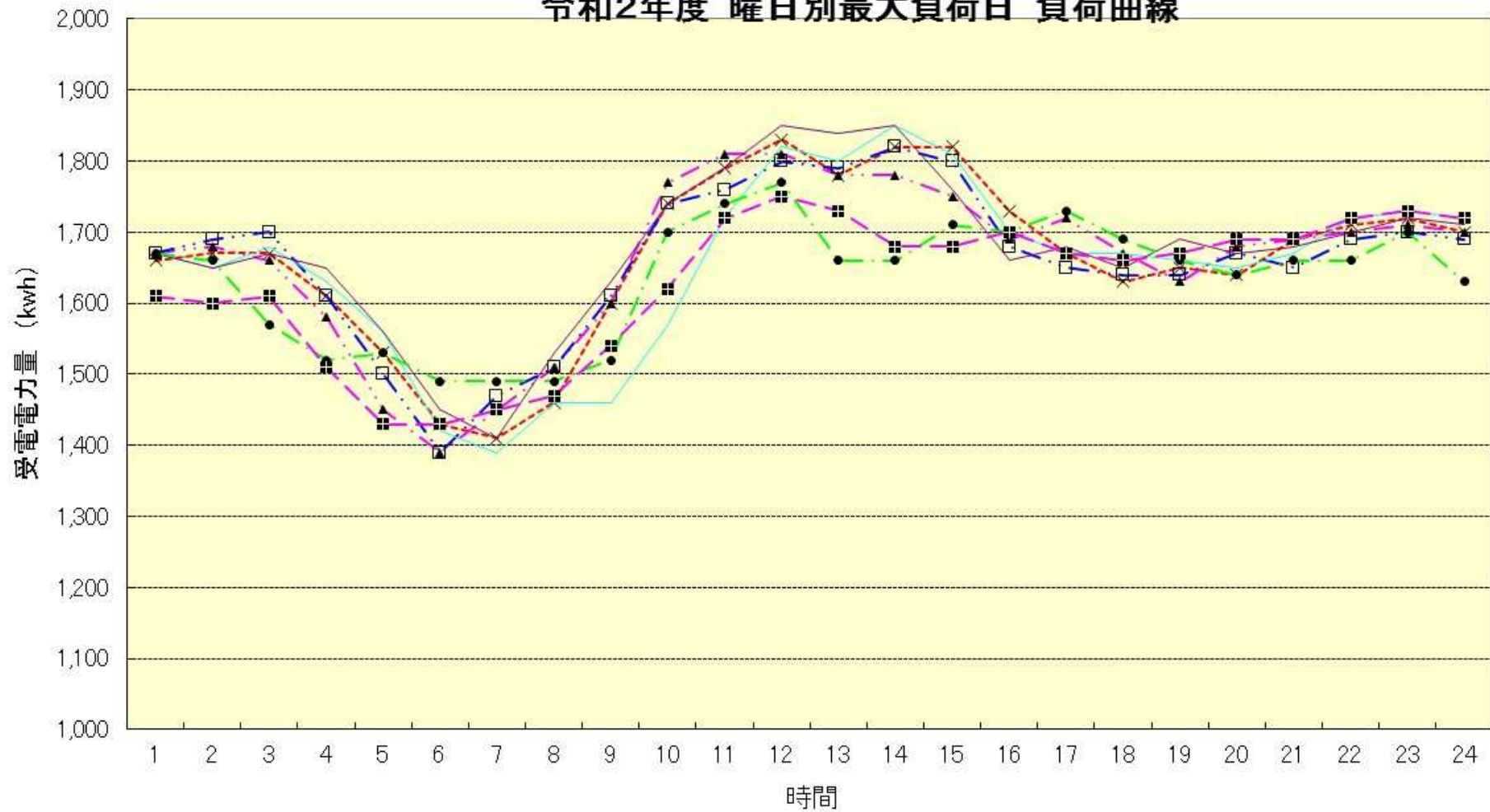
令和2年度 曜日別最大負荷日 負荷曲線
