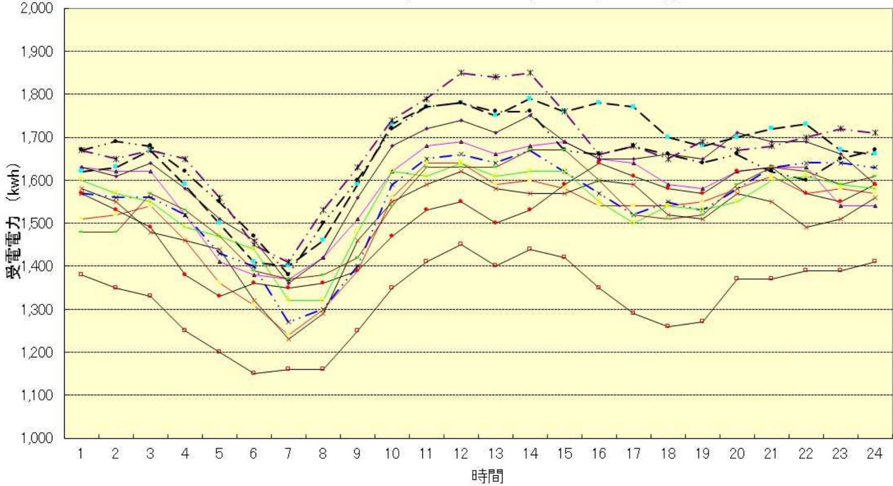
令和2年度 月別最大負荷日負荷曲線
