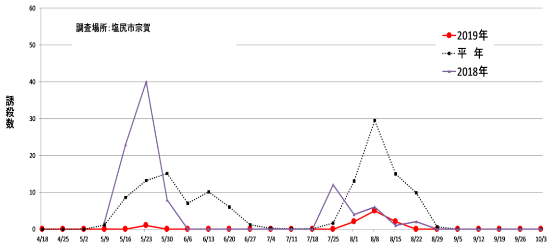
図2 アメリカシロヒトリの誘殺消長（塩尻市宗賀）
