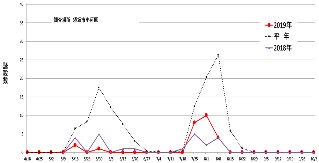
図1 アメリカシロヒトリの誘殺消長（須坂市小河原）
