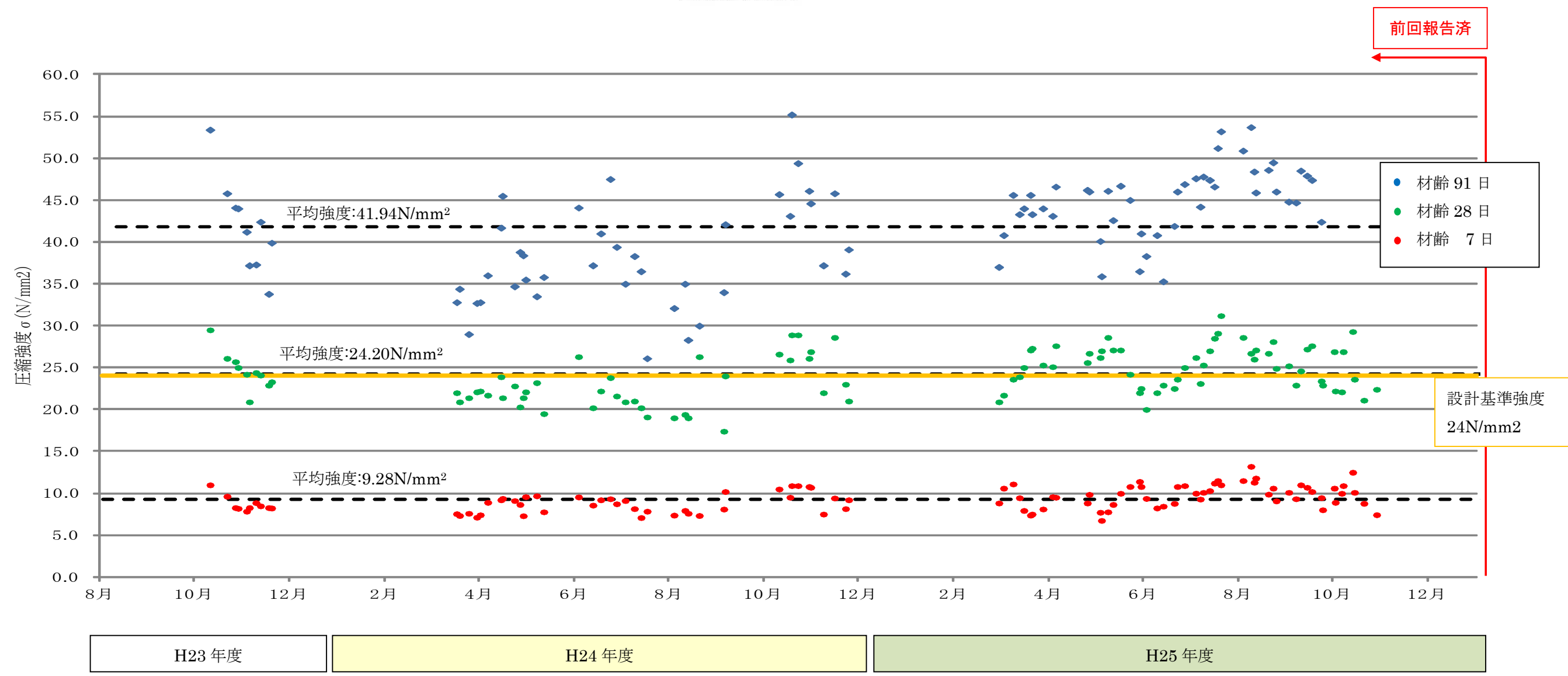
図 3.4.23 コンクリートの圧縮強度の品質管理結果(C3 配合)
