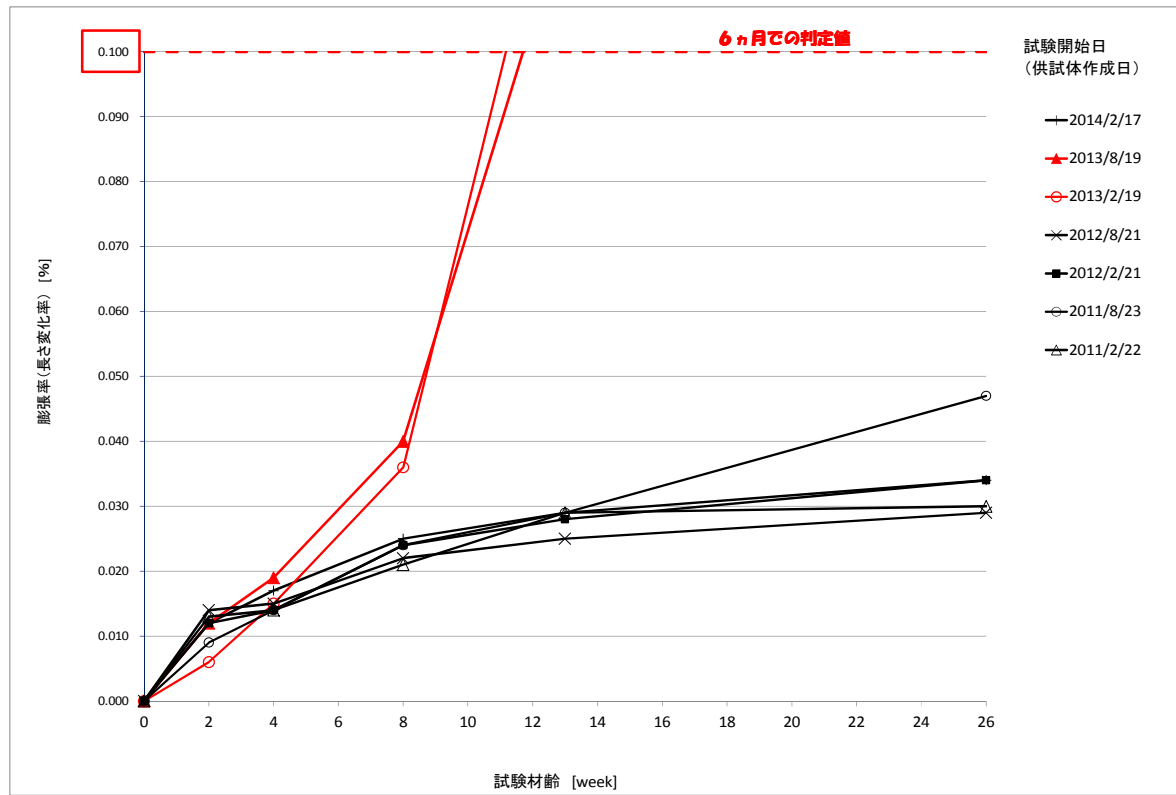
図 3.4.10 アルカリシリカ反応性試験(モルタルバー法)結果
