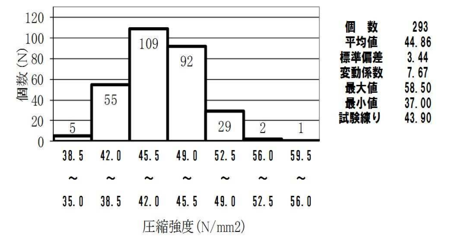
C1配合 圧縮強度ヒストグラム (材齢91日)
