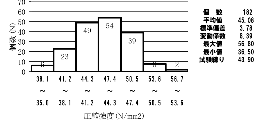
C4配合 圧縮強度ヒストグラム (材齢91日)
