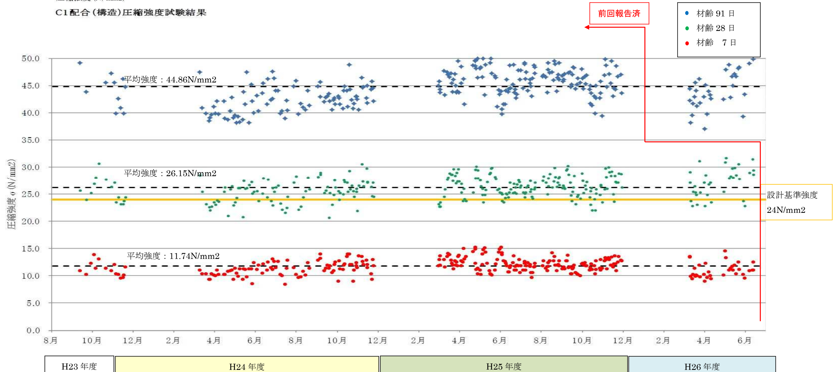
図 3.4.21 コンクリートの圧縮強度の品質管理結果(C1 配合)
