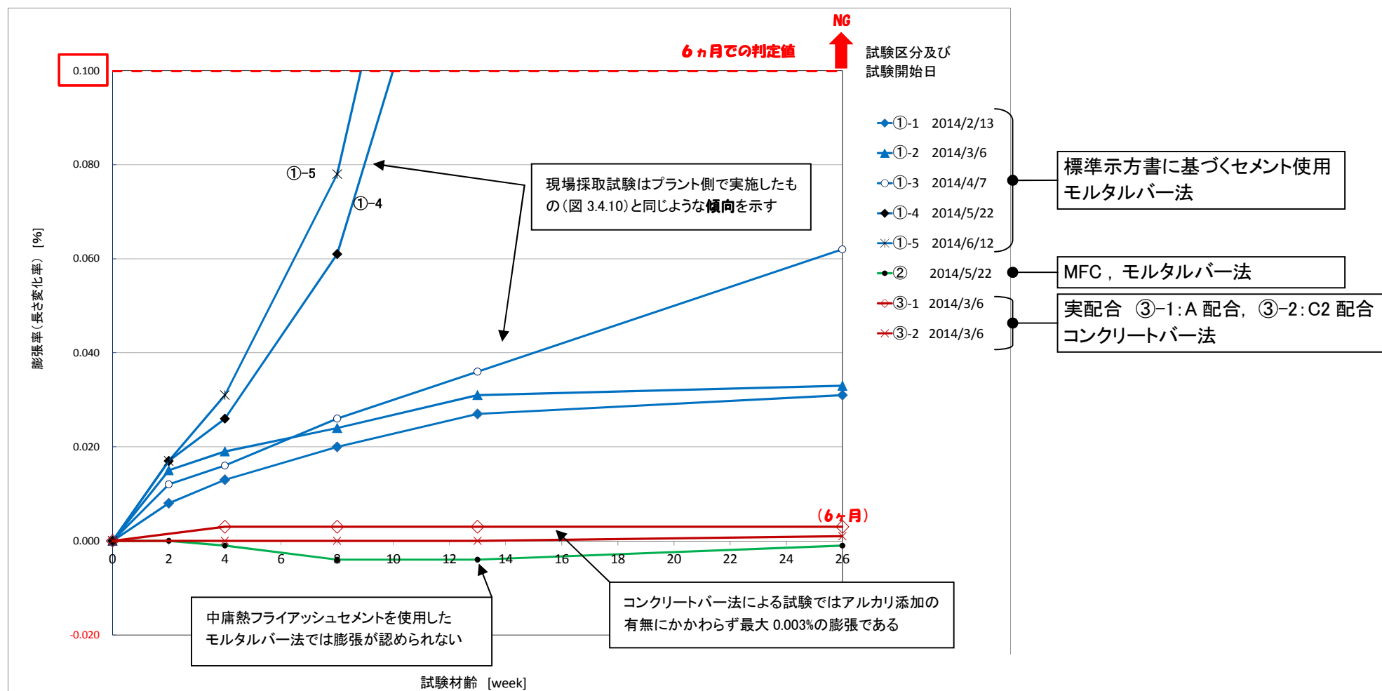
図 3.4.12 追加試験結果
