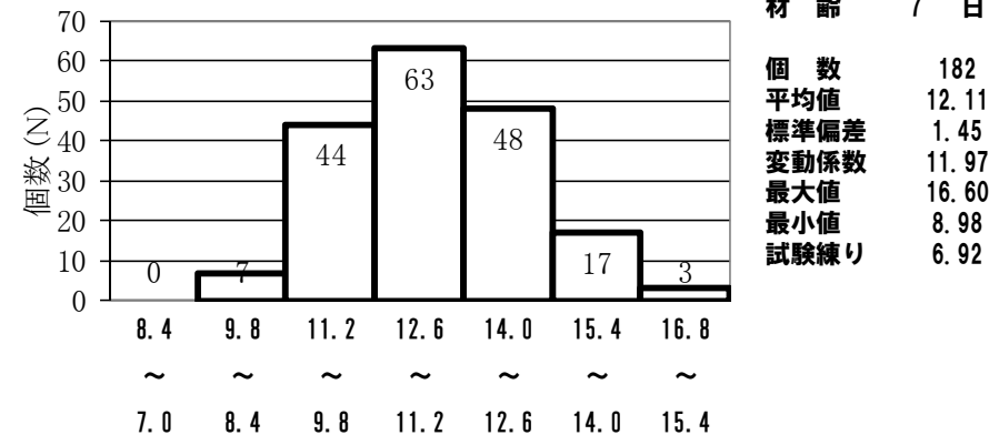
C4配合 圧縮強度ヒストグラム (材齢7日)
