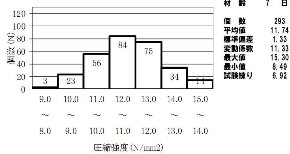
C1配合(構造)圧縮強度試験結果
