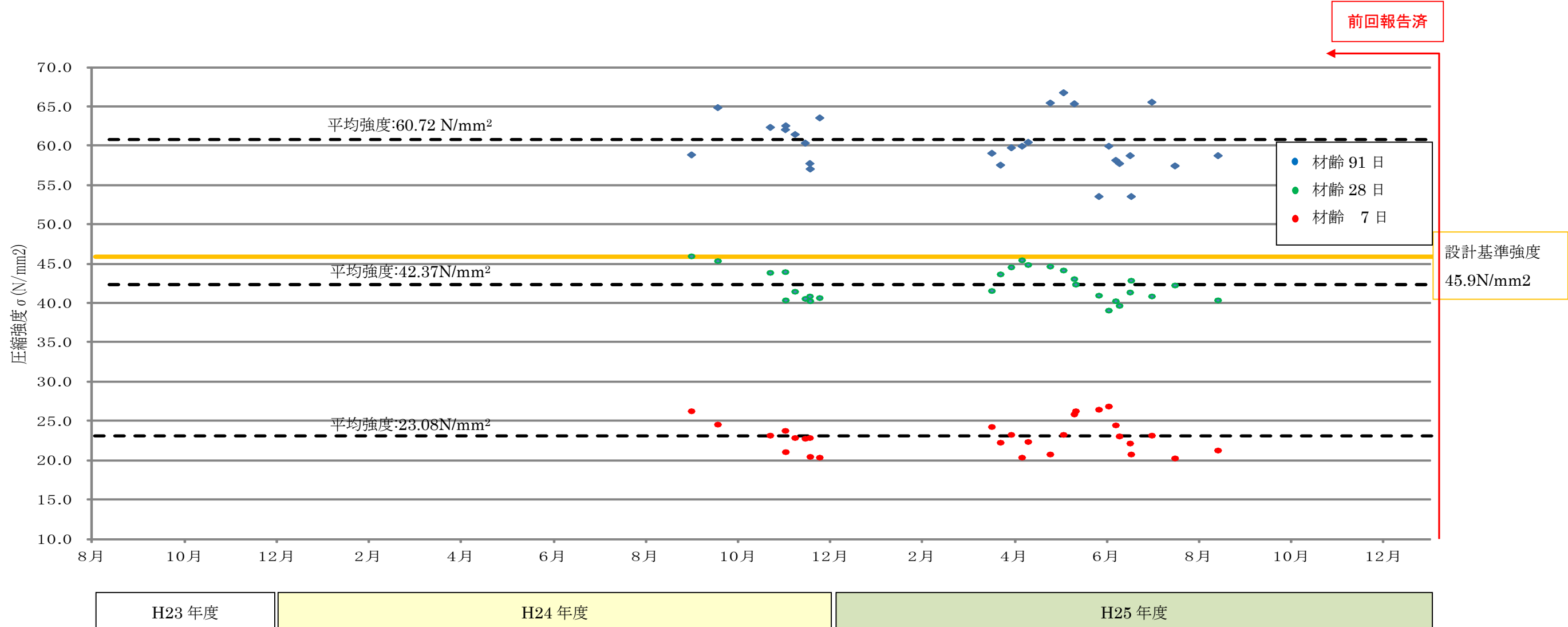
図 3.4.22 コンクリートの圧縮強度の品質管理結果(C2 配合)
