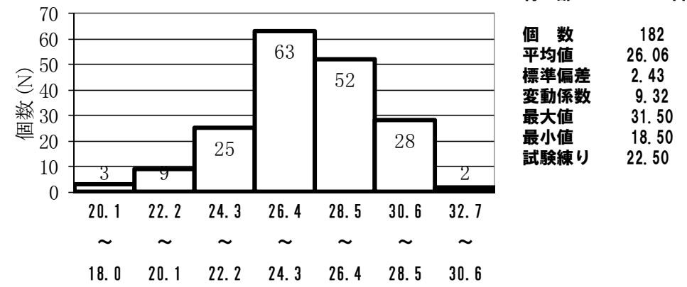
C4配合 圧縮強度ヒストグラム (材齢28日)
