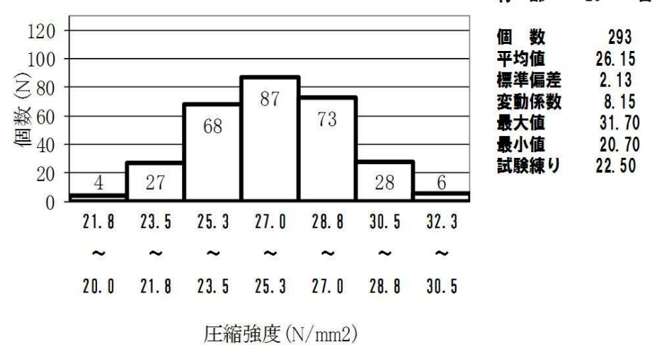
C1配合 圧縮強度ヒストグラム (材齢28日)
