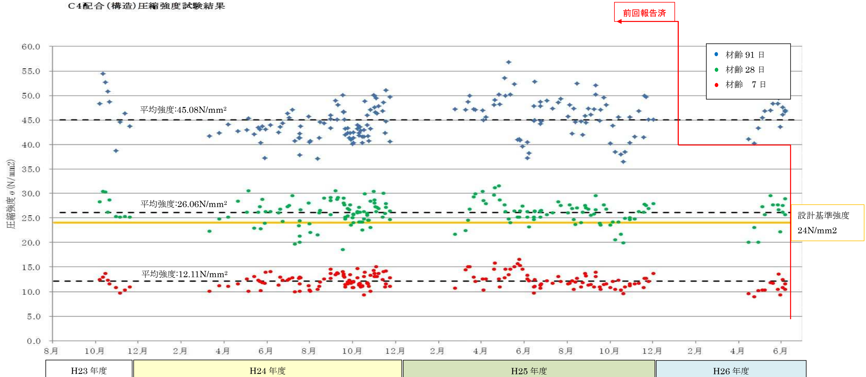
図 3.4.24 コンクリートの圧縮強度の品質管理結果(C4 配合)
