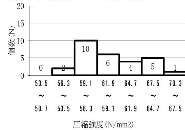
C2配合 圧縮強度ヒストグラム (材齢91日)
