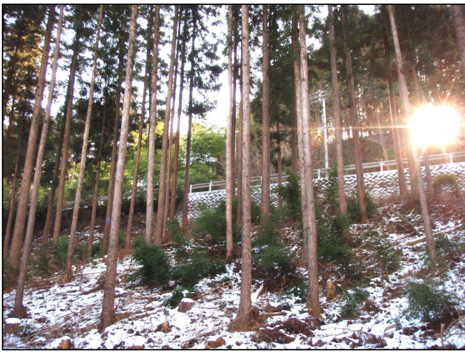
《間伐奨励賞》 飯伊森林組合阿智支所 肥後班 作業路から間伐材を直接プロセッサでつかんで造材し、生産性を向上させました。間伐と併せ、林内に侵入した竹を整理したことで、林内環境を大きく改善しています。
