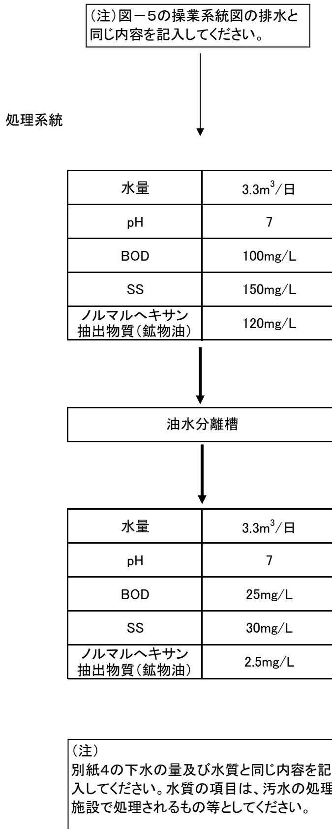
図-7 汚水処理の系統図
