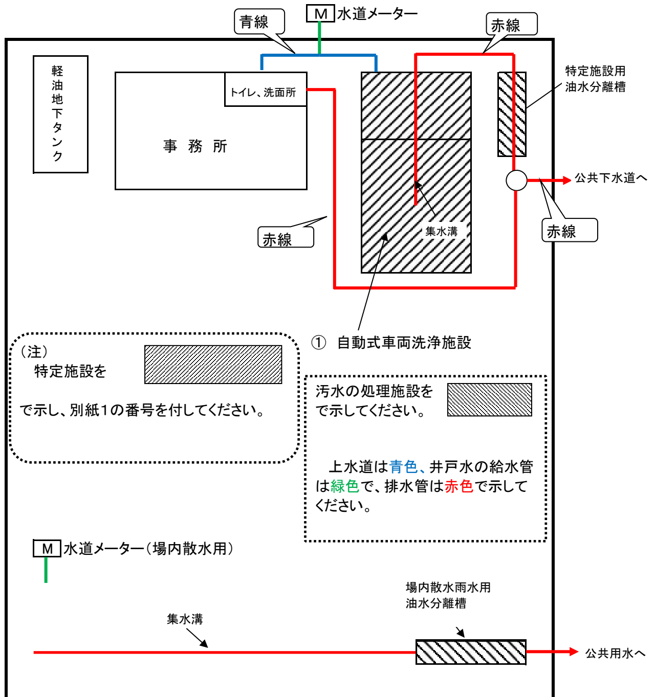
図-3 特定施設等主要機器の配置図
