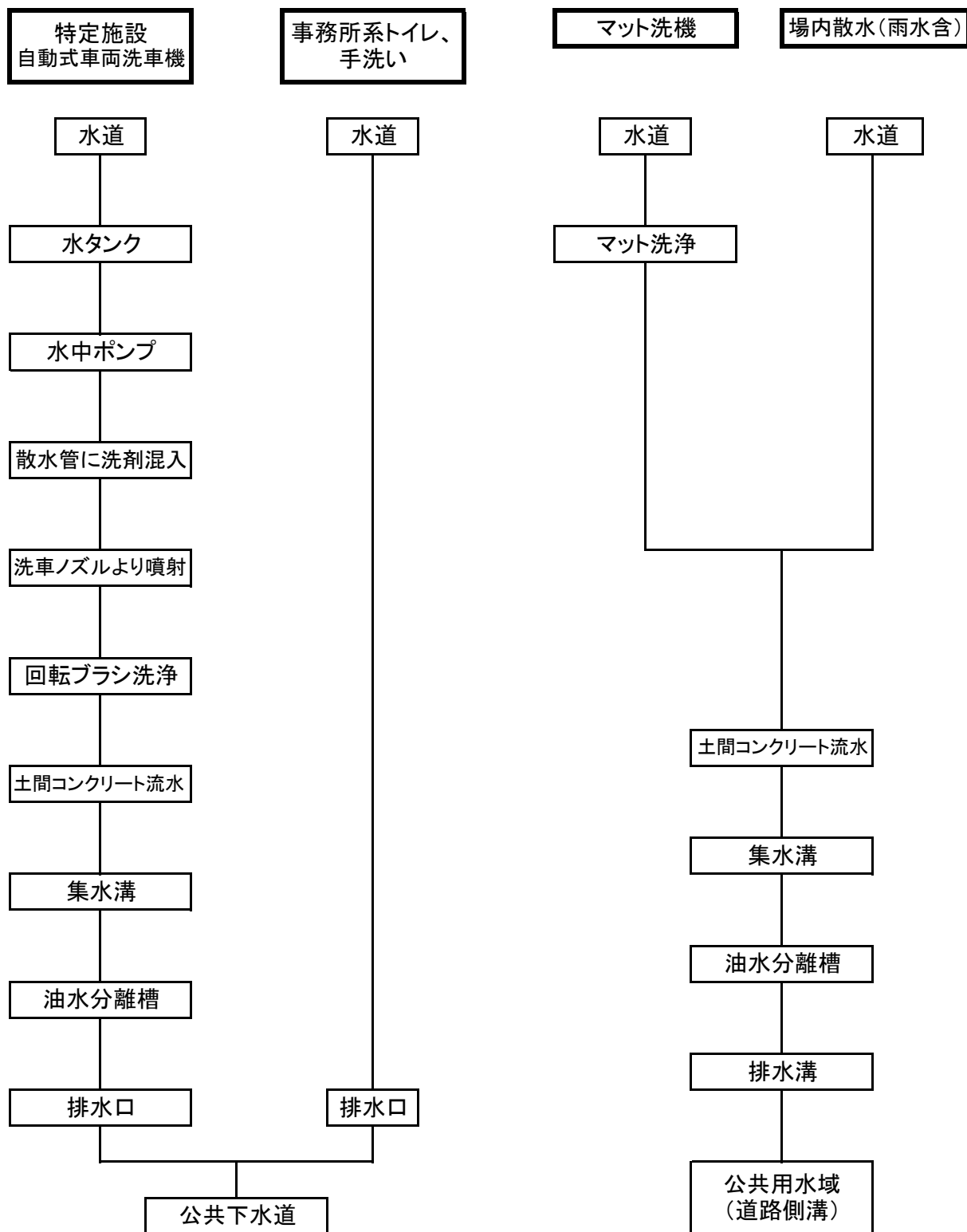
図-5 特定施設の操業系統図
