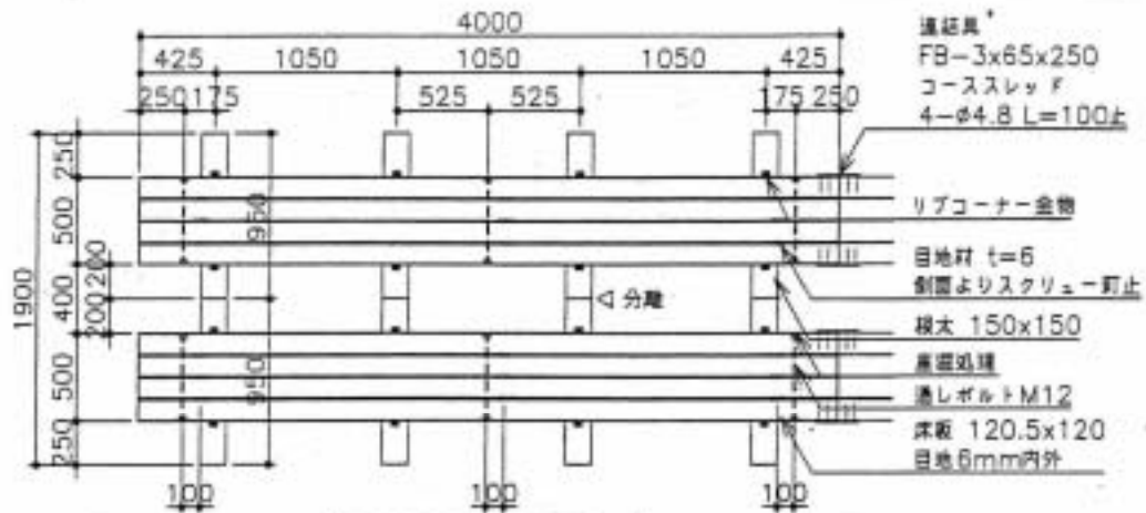
平面図 S=1:40
