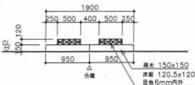
断面図 S=1:40
