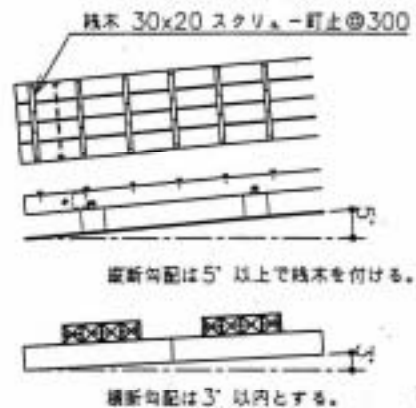
勾配参考図 S=1:40
