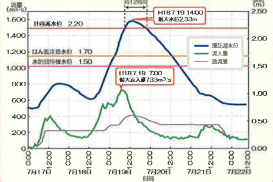
諏訪湖の水位と流入放流量
