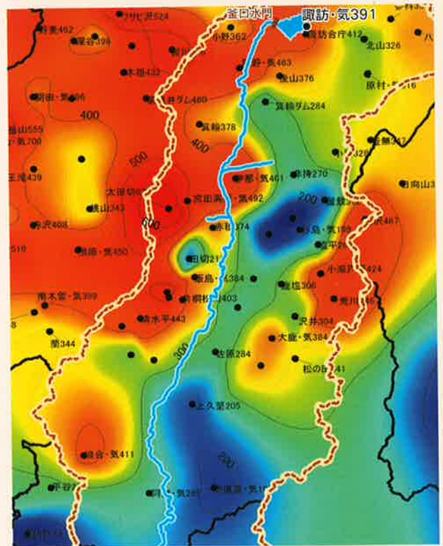
雨量地域分布 (H18. 7. 15~21)
