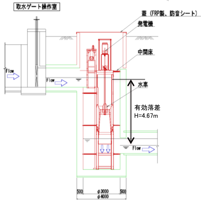
発電設備概要
