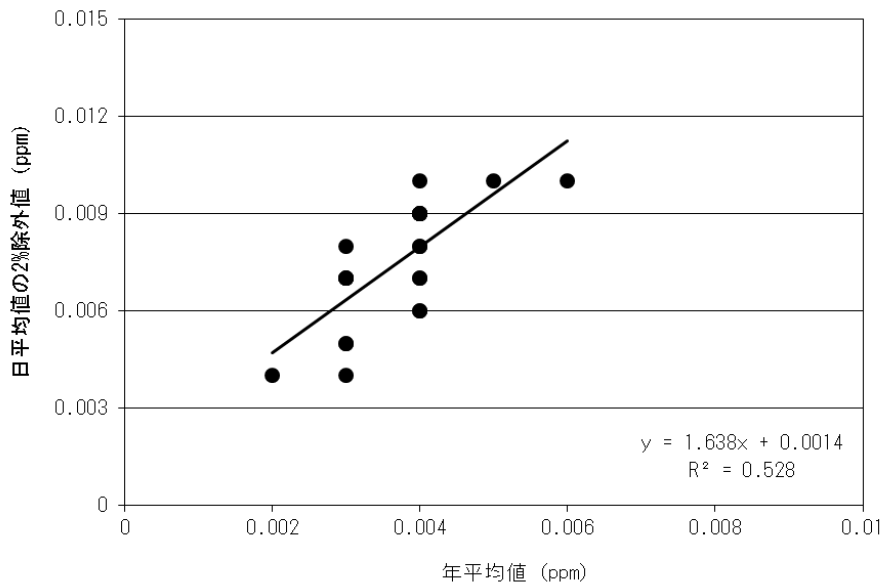
図2.5-1(1) 日平均値の2%除外値への変換式（二酸化硫黄）
