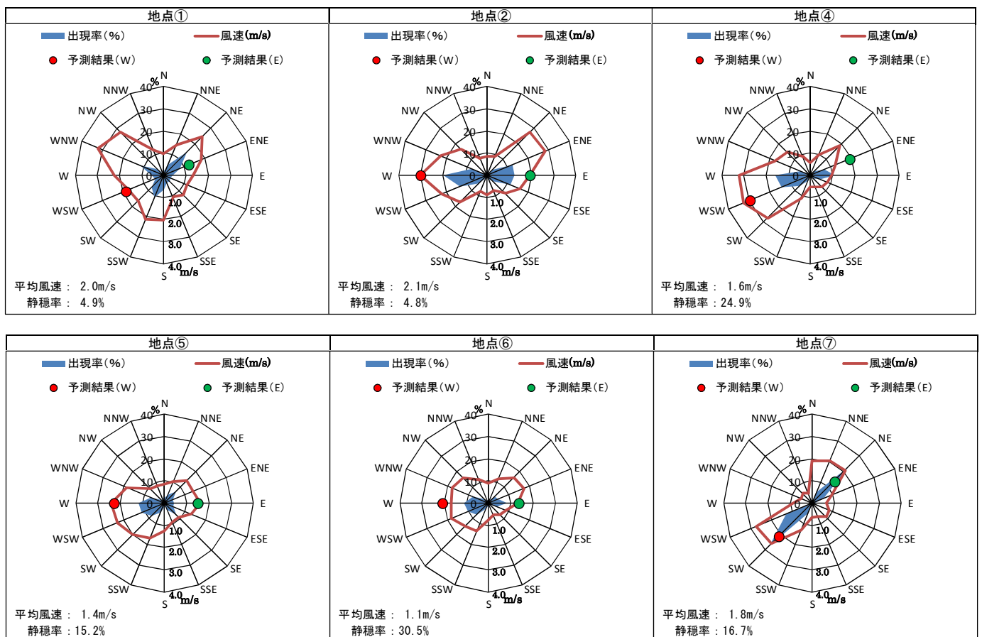
図2.3-1(1) 風の場の予測結果 (1/2)
