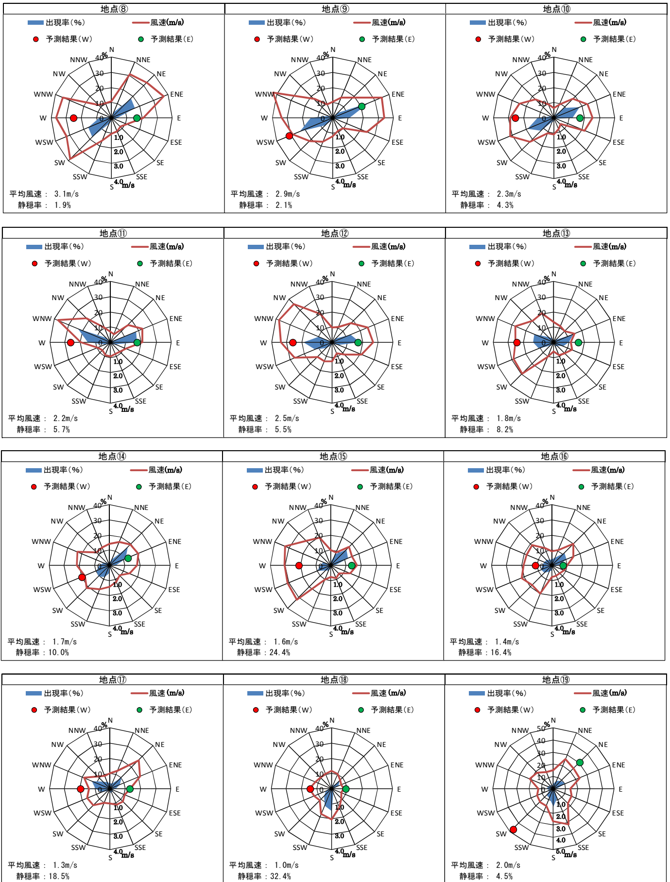
図2.3-1(2) 風の場の予測結果 (2/2)
