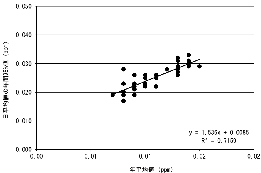
図2.5-1(2) 日平均値の年間98%値への変換式（二酸化窒素）
