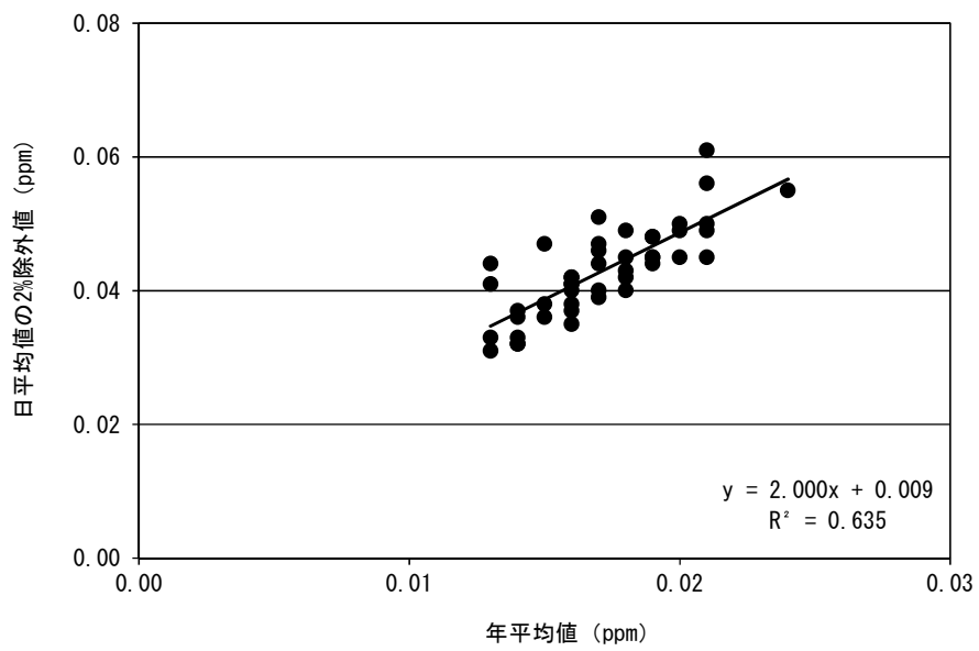
図2.5-1(3) 日平均値の2%除外値への変換式 (浮遊粒子状物質)
