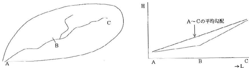
図1-5 クラーヘン式の勾配区分
