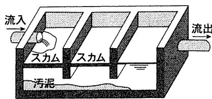
沈殿分離槽
