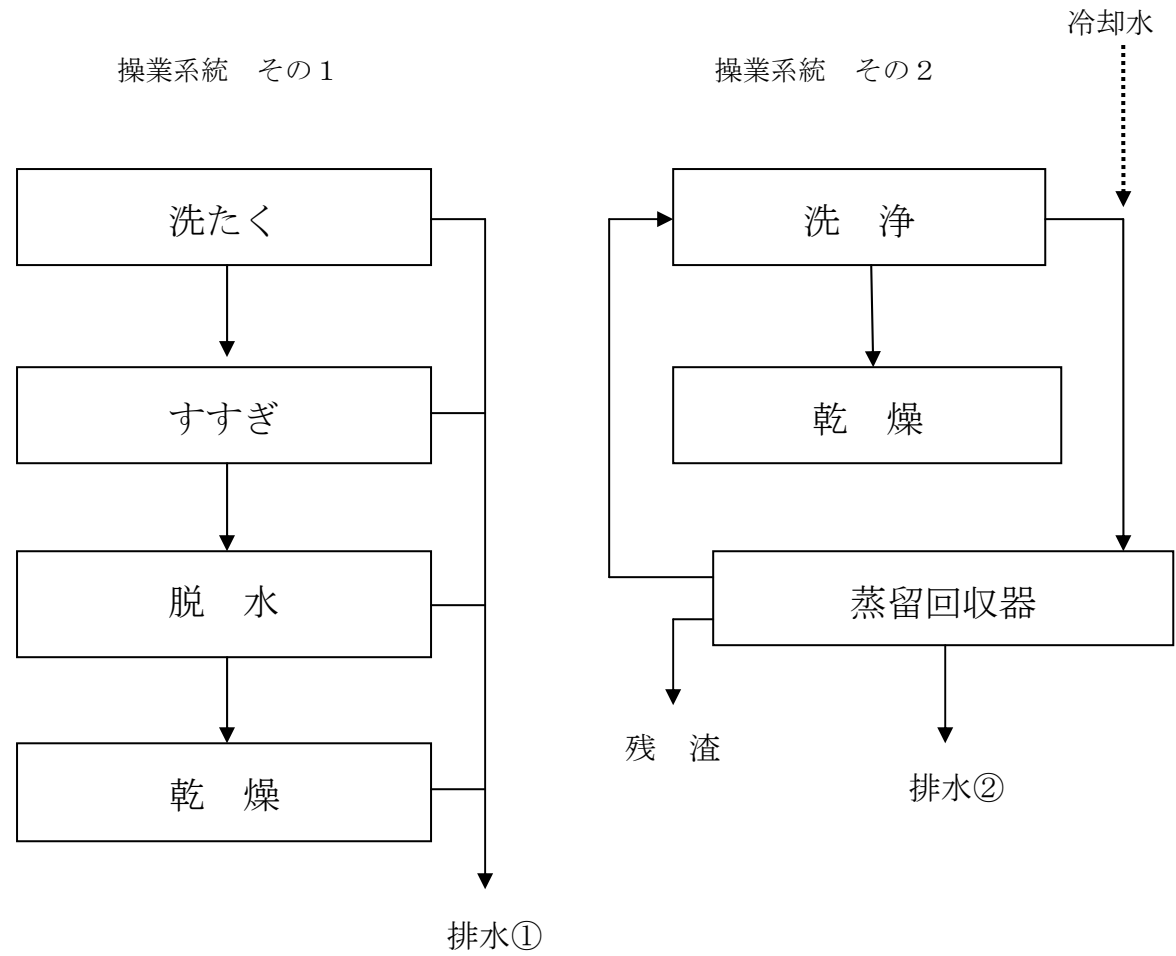
図—5 特定施設の作業系統図
