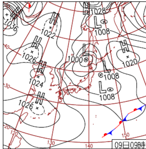
図 1-9 地上天気図（2月9日）
