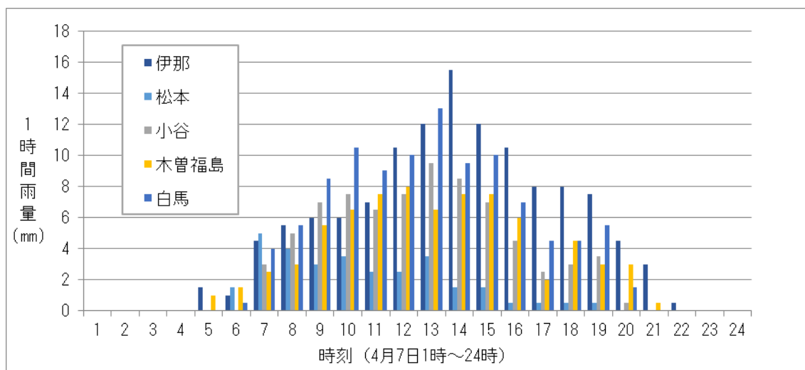
図 3-2 各地の雨量変化（4月7日）
