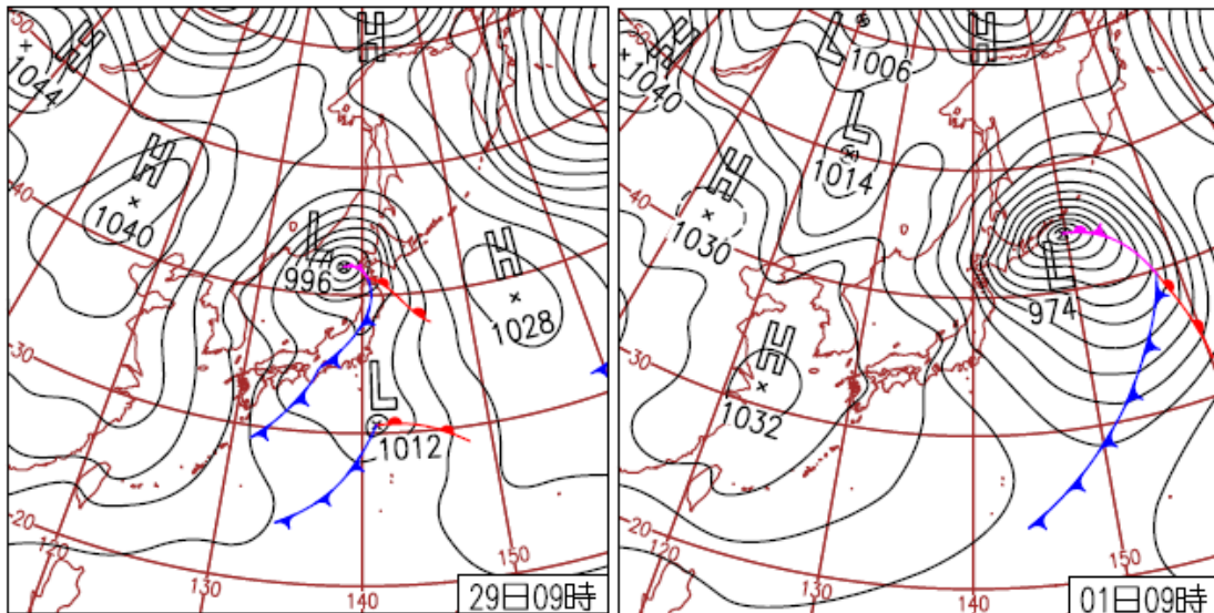
図1-13 地上天気図（2月29日～3月1日）
