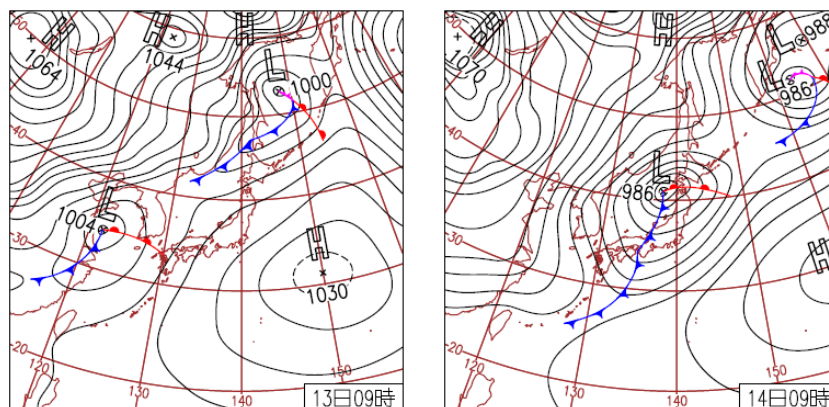
図 2-1 地上天気図（2月13日～2月14日）
