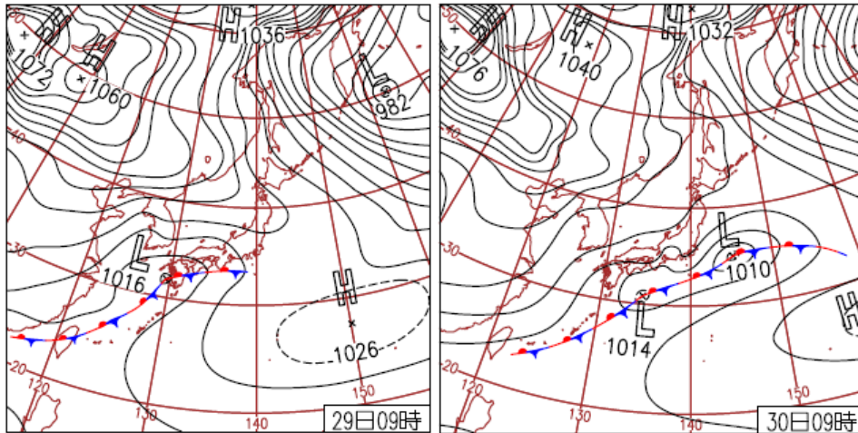
図1-7 地上天気図（1月29日～1月30日）
