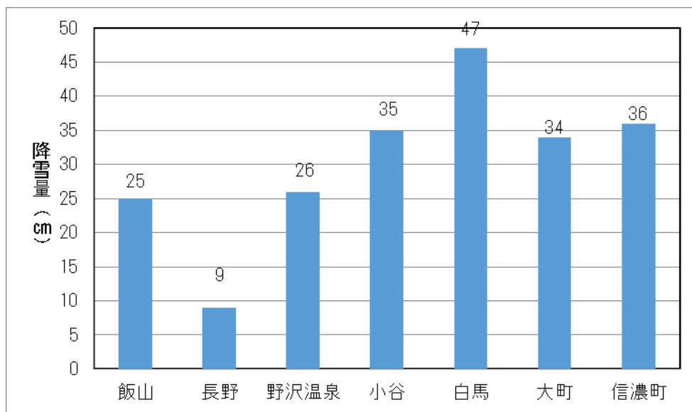
図 1-10 各地の降雪量（2月9日）
