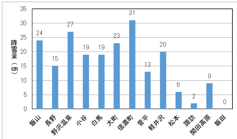
図1-8 各地の降雪量（1月29日～1月30日）
