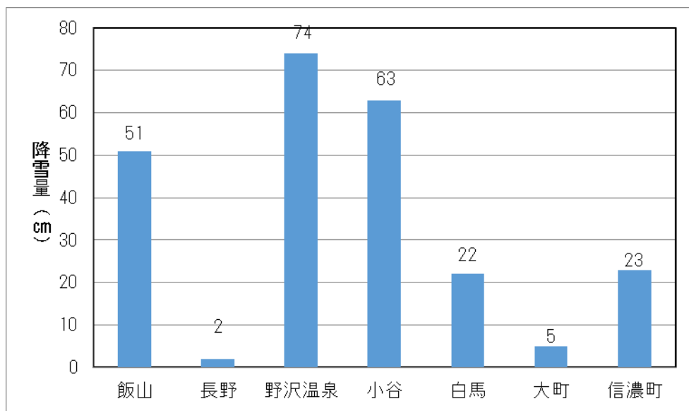
図 1-12 各地の降雪量（2月15日～2月17日）
