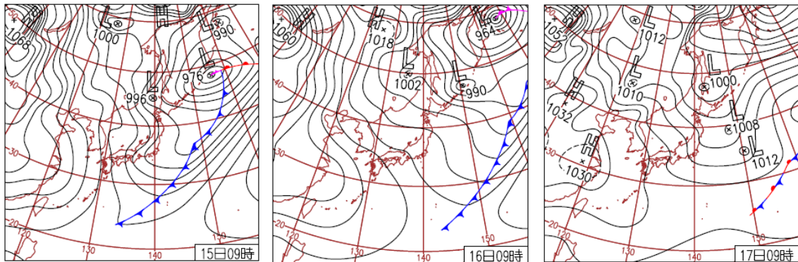
図 1-11 地上天気図（2月15日～2月17日）
