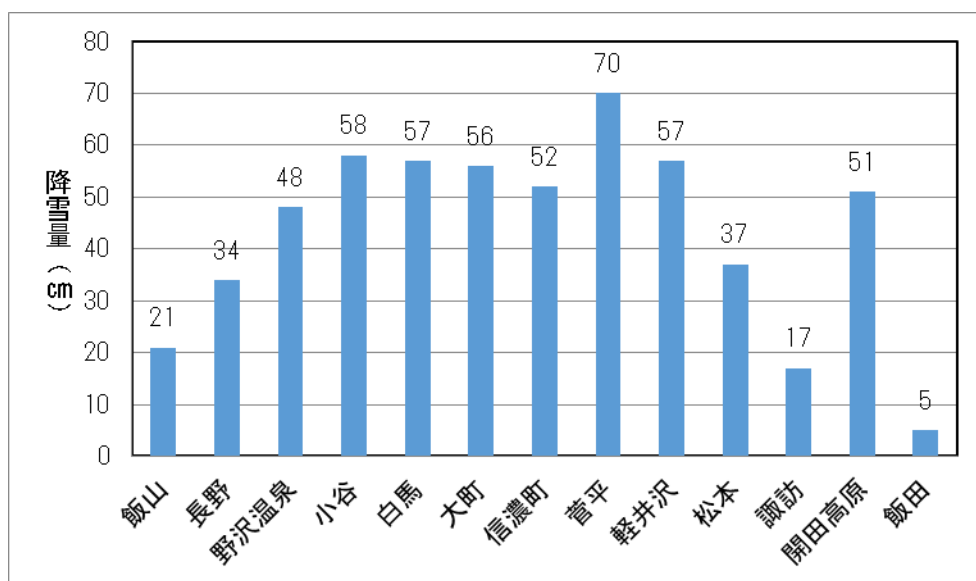
図 1-4 各地の降雪量（1月18日～1月20日）
