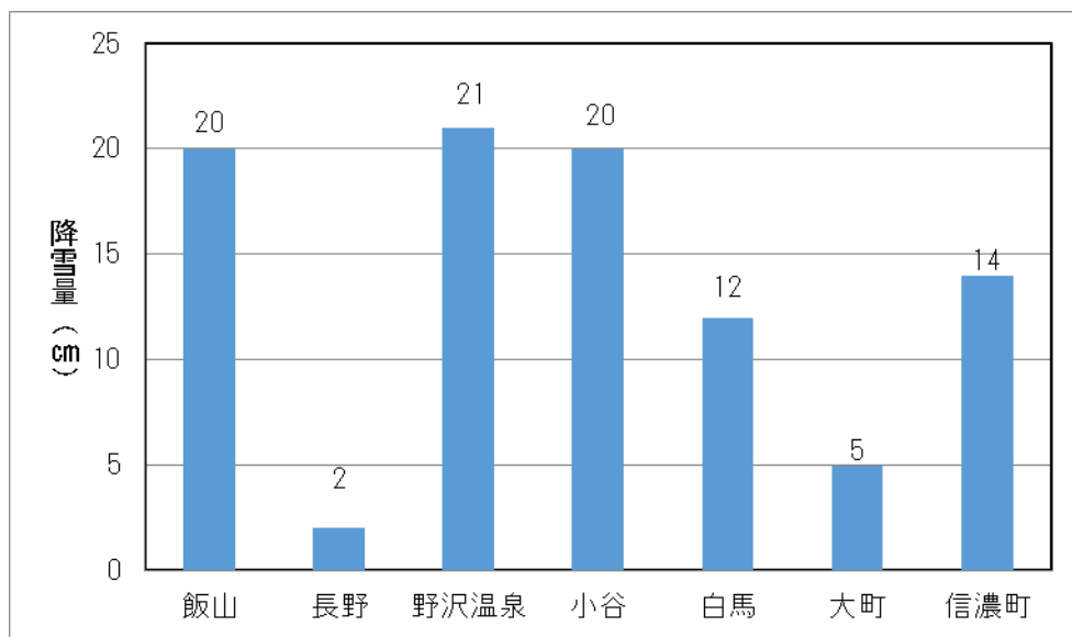
図 1-6 各地の降雪量（1月24日）
