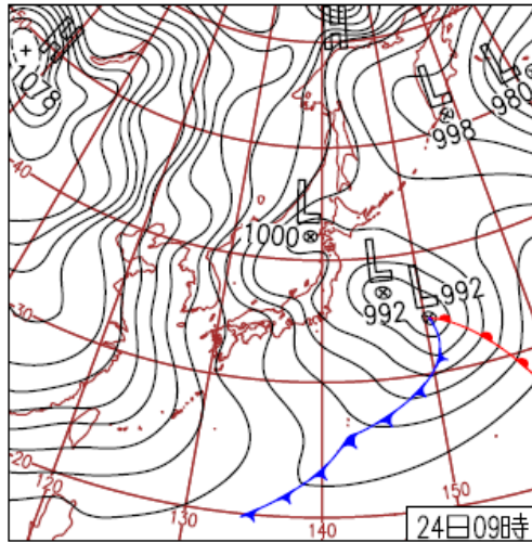
図 1-5 地上天気図（1月24日）
