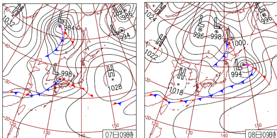
図 3-1 地上天気図（4月7日～4月8日）
