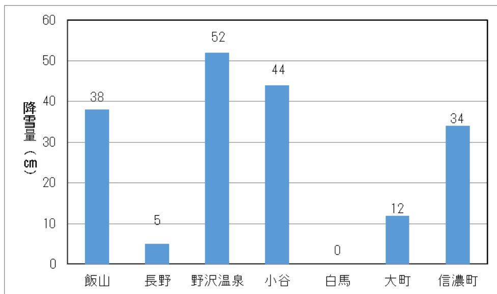
図1-14 各地の降雪量（2月29日～3月1日）
