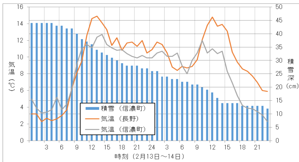
図 2-2 長野・信濃町の気温と積雪の変化（2月13日～14日）
