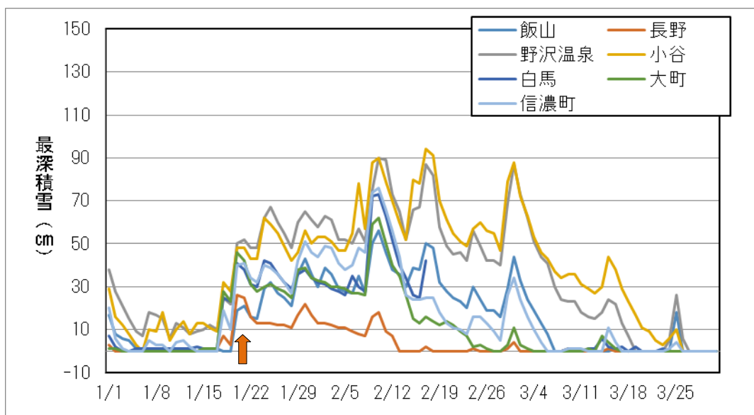
図 1-2 各地の最深積雪（1月1日～3月31日）
