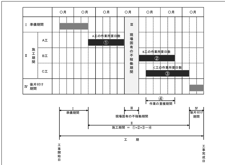
図1 工程表
