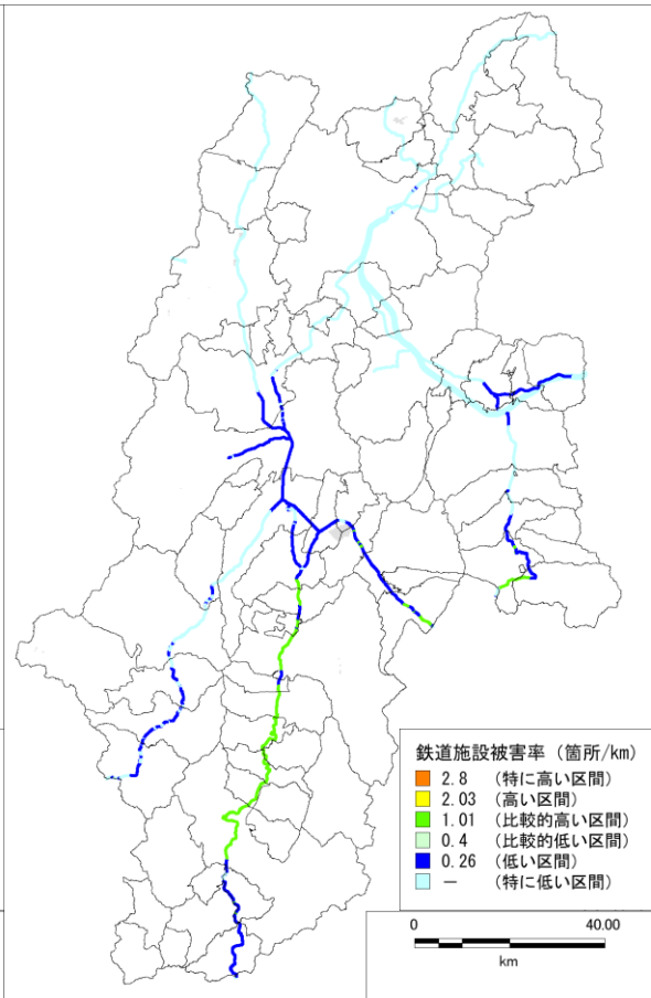
図 5.2-11 南海トラフ巨大地震（基本ケース）における鉄道施設被害率分布図
