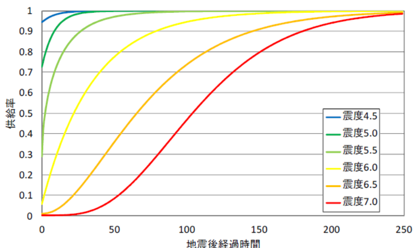
図 7.1-4 電力の計測震度に対する供給率曲線の予測
