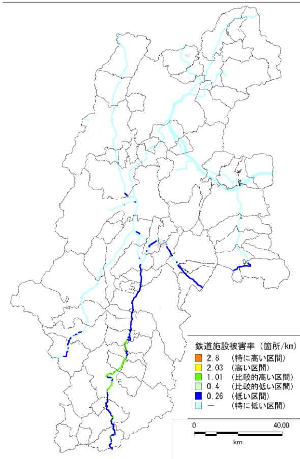
図 5.2-10 想定東海地震における鉄道施設被害率分布図
