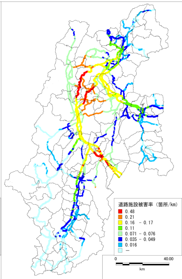
図 5.1-3 糸魚川-静岡構造線断層帯の地震(全体)における道路施設被害率分布図
