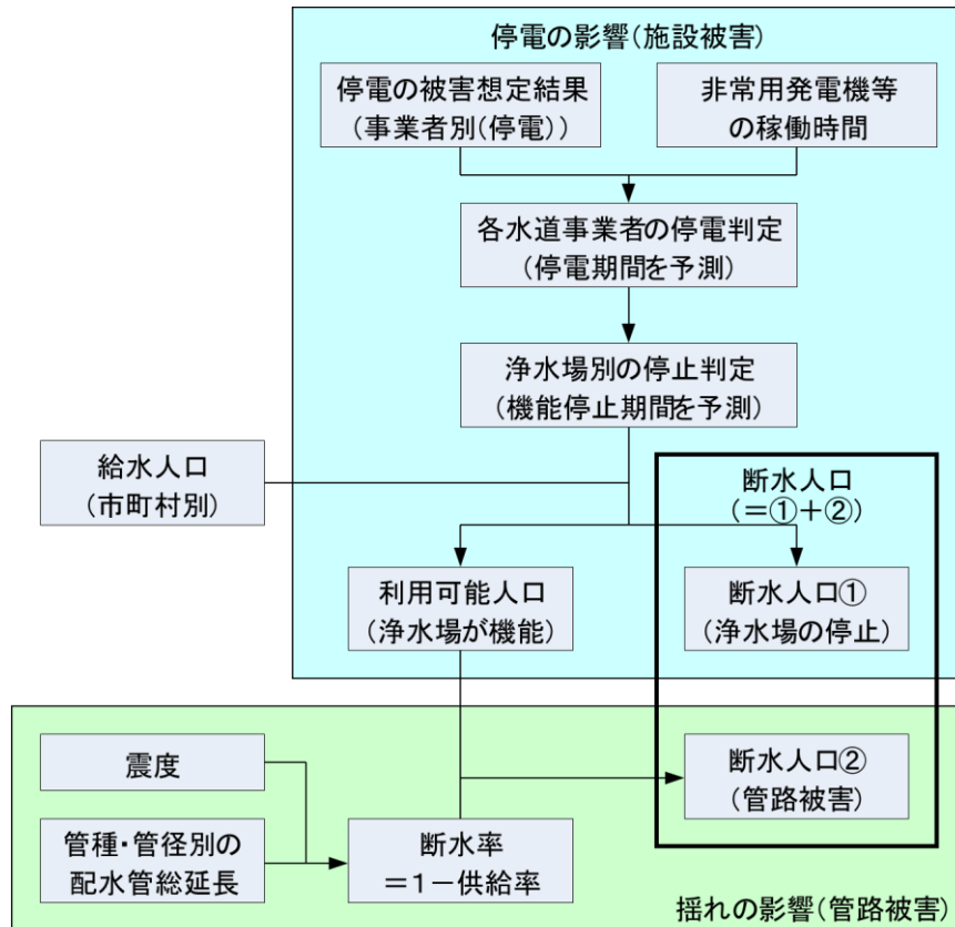
図 6.1-2 断水人口の算定フロー
