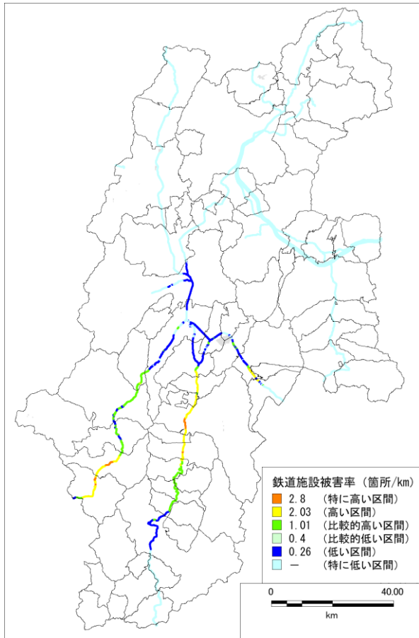
図 5.2-8 木曾山脈西縁断層帯(主部北部)の地震(ケース1)における鉄道施設被害率分布図
