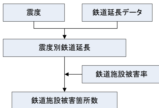
図 5.2-1 鉄道施設被害箇所数の算定フロー
