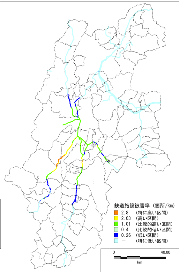
図 5.2-9 境峠・神谷断層帯(主部)の地震(ケース1)における鉄道施設被害率分布図
