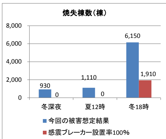
図 1. 2. 2-2 今回の被害想定結果及び感震ブレーカー設置率 100%時の焼失棟数比較 ※重複処理後の全壊棟数で比較
