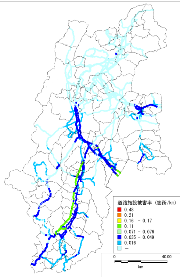
図 5.1-11 南海トラフ巨大地震（基本ケース）における道路施設被害率分布図
