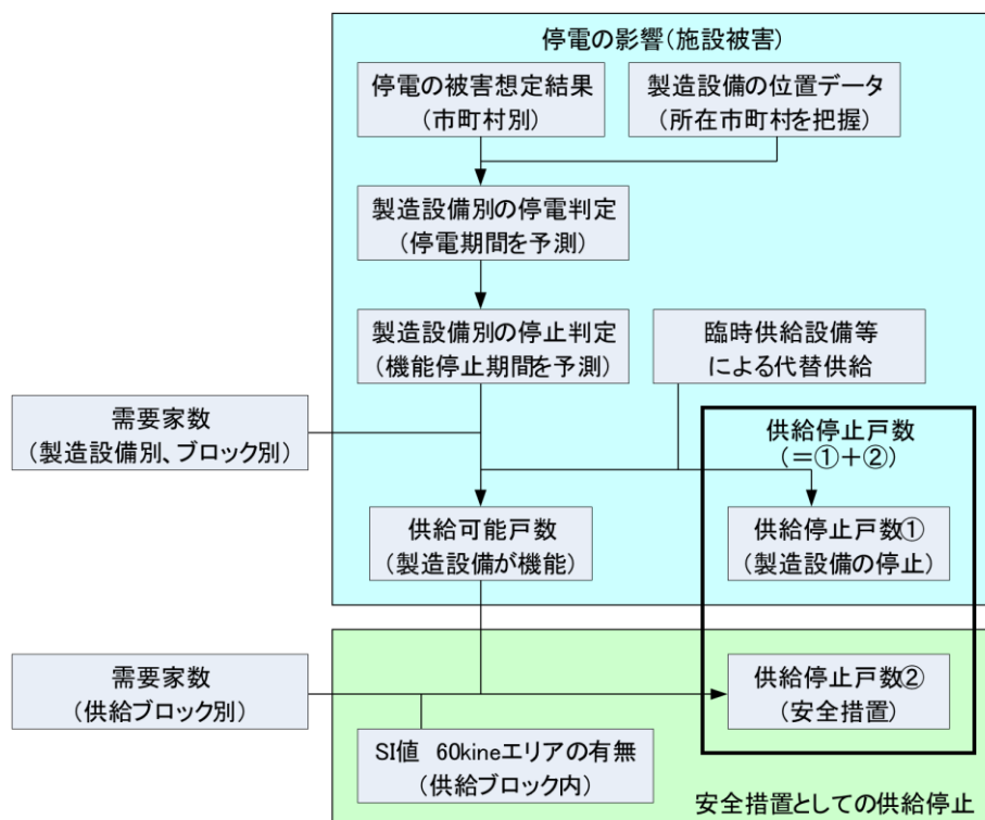
図 6.3-2 供給停止戸数の算定フロー
