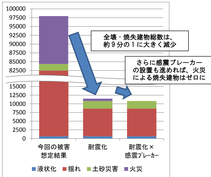
図 1. 4. 1-2 今回の被害想定結果、耐震化率 100%、耐震化率 100%×感震プレーカー設置率 100%の場合の全壊・焼失建物数
