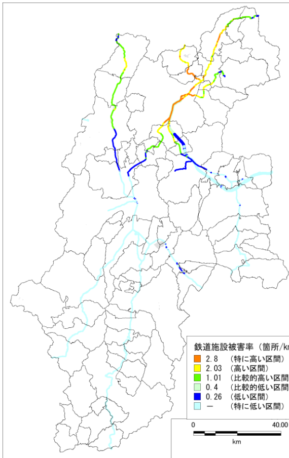
図 5.2-2 長野盆地西縁断層帯の地震(ケース 3)における鉄道施設被害率分布図
