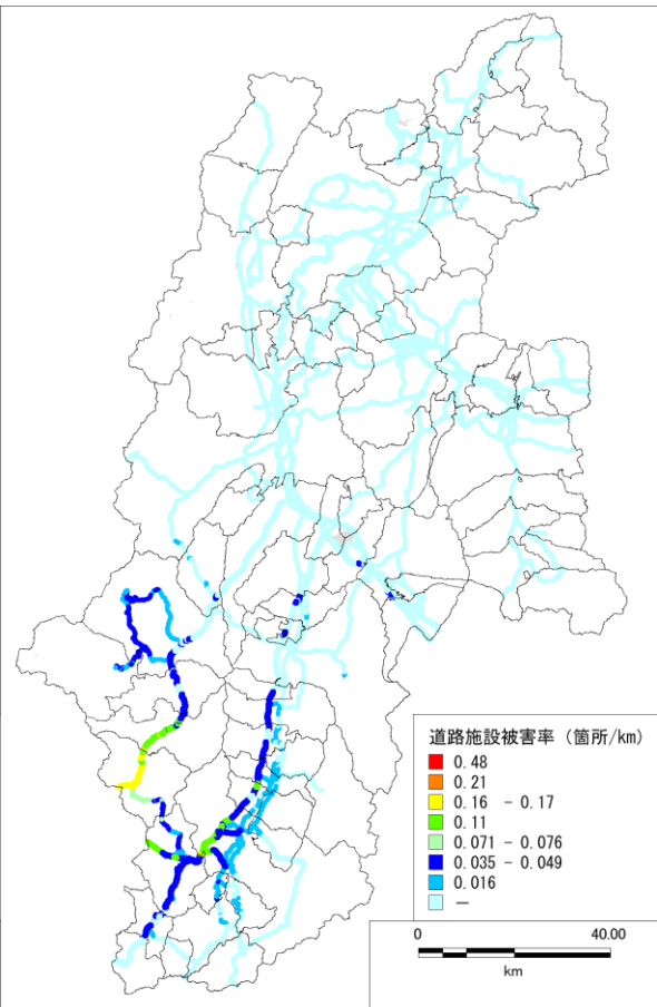
図 5.1-7 阿寺断層帯（主部南部）の地震（ケース 1）における道路施設被害率分布図
