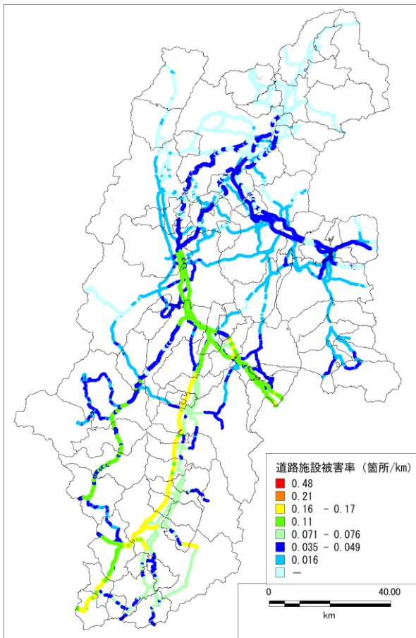
図 5.1-12 南海トラフ巨大地震（陸側ケース）における道路施設被害率分布図
