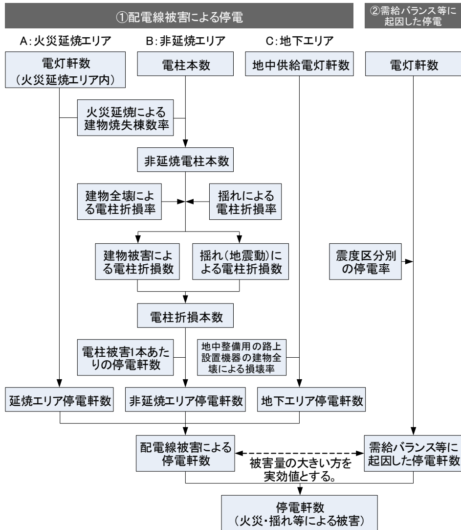
図 6.4-3 停電軒数の算定フロー
