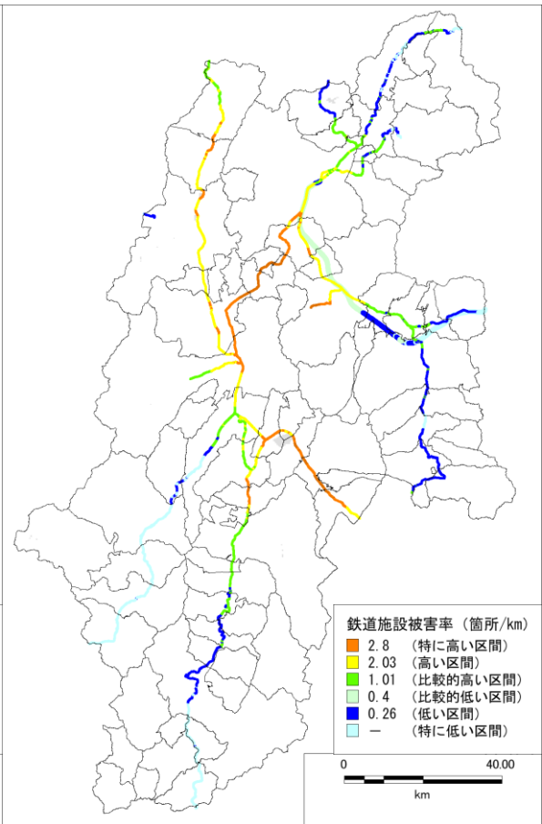
図 5.2-3 糸魚川-静岡構造線断層帯の地震(全体)における鉄道施設被害率分布図
