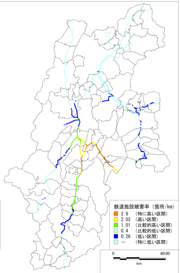
図 5.2-5 糸魚川-静岡構造線断層帯の地震(南側)における鉄道施設被害率分布図
