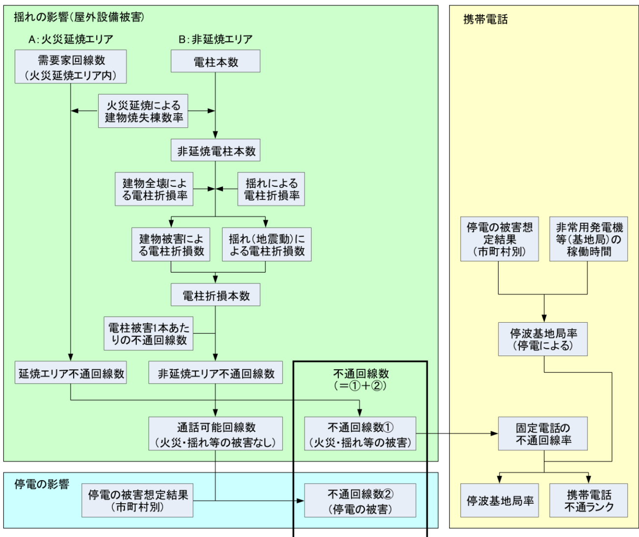
図 7.1-3 不通回線数、携帯電話不通ランクの算定フロー
