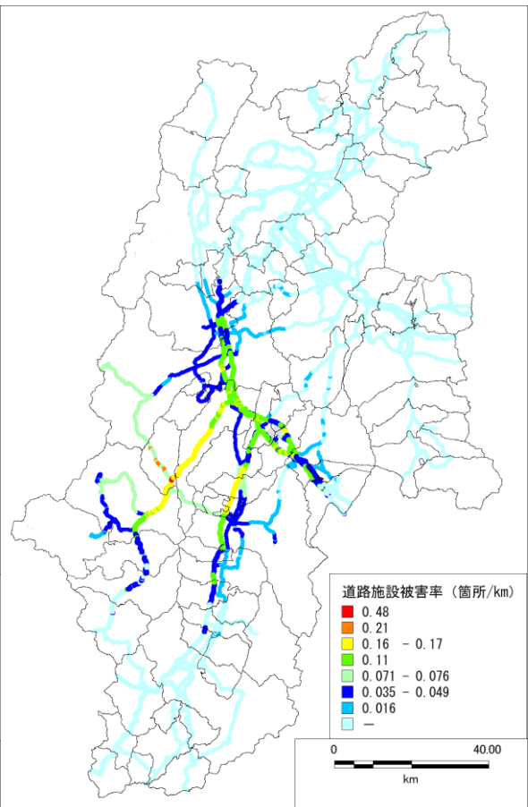
図 5.1-9 境峠・神谷断層帯（主部）の地震（ケース 1）における道路施設被害率分布図
