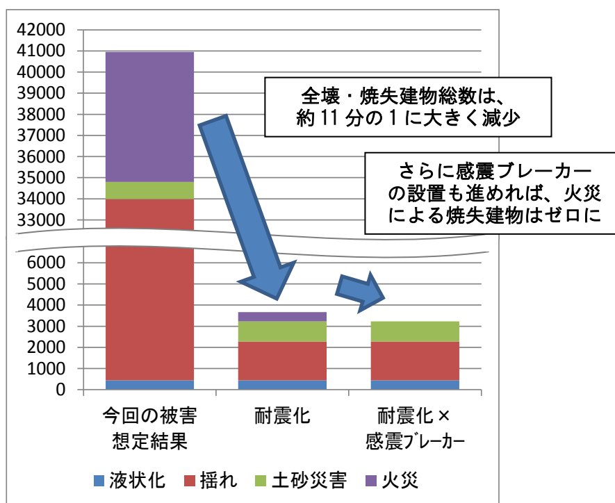
図 1.4.1-1 今回の被害想定結果、耐震化率 100%、耐震化率 100% × 感震プレーカー設置率 100% の場合の全壊・焼失建物数
