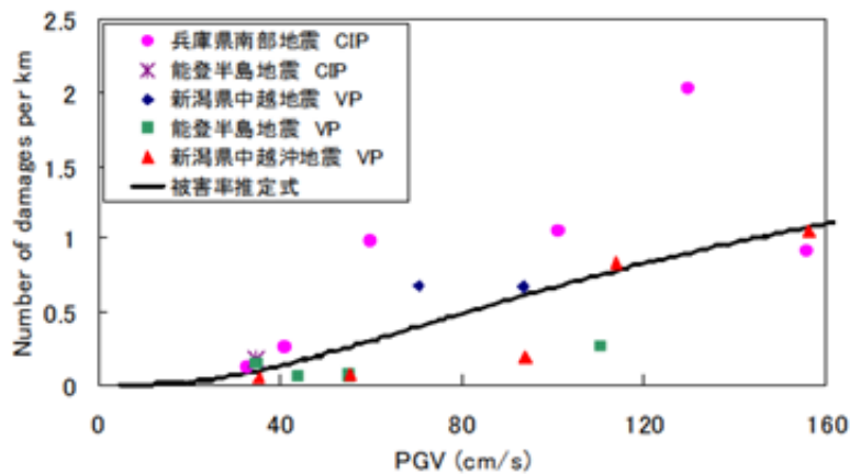
図 6.1-3 基準被害率(箇所/km) (丸山・山崎, 2009)
