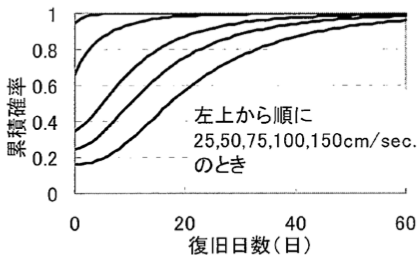
図 6.2-3 下水道の供給率復旧曲線（日下ほか, 2011）
