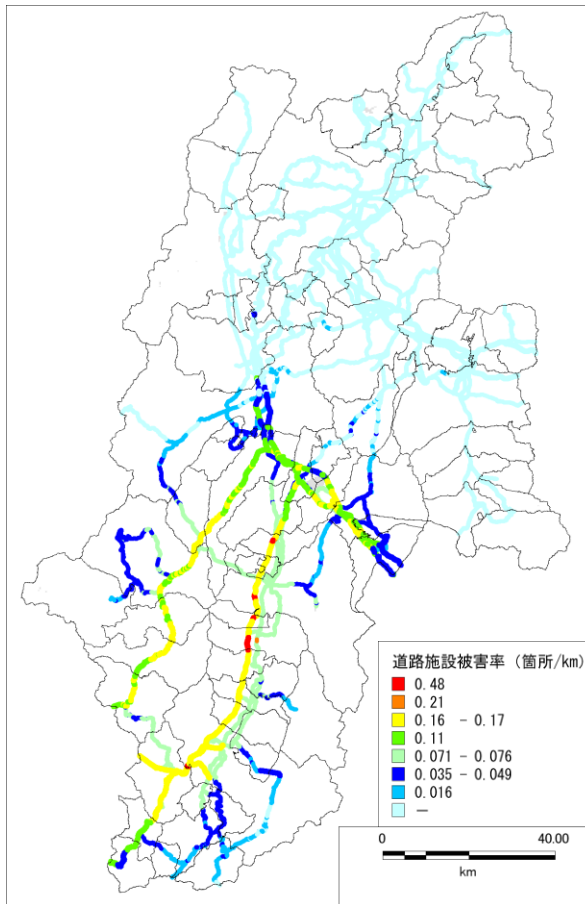
図 5.1-6 伊那谷断層帯（主部）の地震（ケース 3）における道路施設被害率分布図
