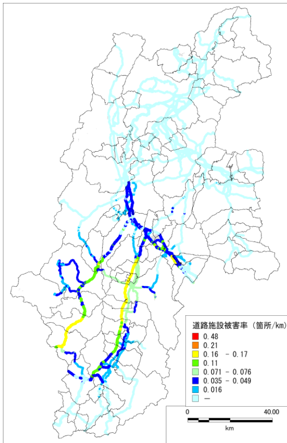
図 5.1-8 木曾山脈西縁断層帯（主部北部）の地震（ケース 1）における道路施設被害率分布図
