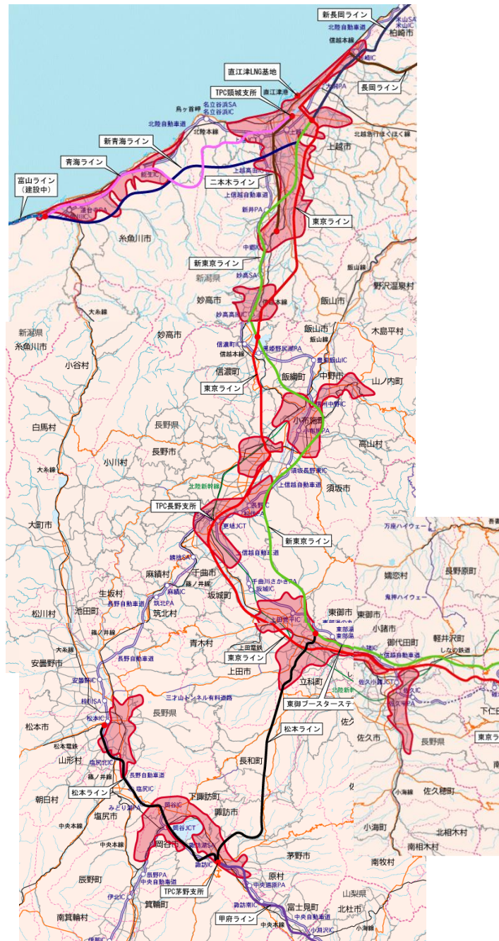
図 6.3-3 主要幹線パイプライン(国際石油開発帝石(株)ホームページより) (—: 東京ライン、—: 新東京ライン、—: 松本ライン、■: 各ガス会社の都市ガス供給地域)
