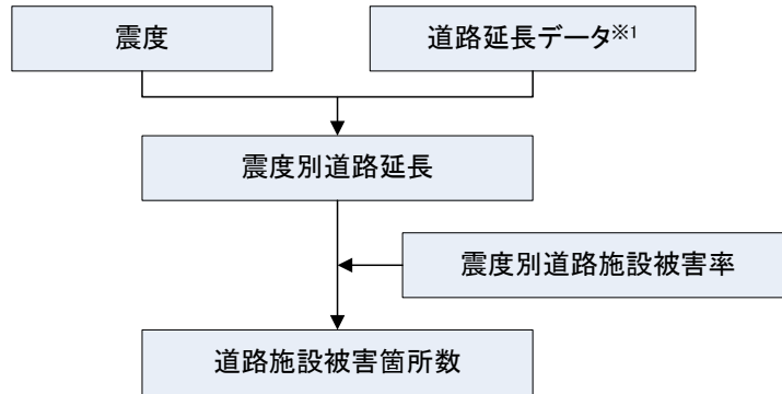
図 5.1-1 道路施設被害箇所数の算定フロー
