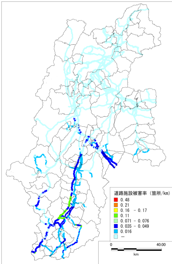
図 5.1-10 想定東海地震における道路施設被害率分布図
