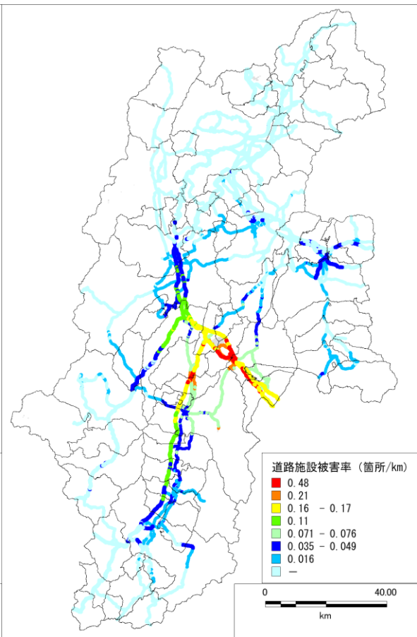
図 5.1-5 糸魚川-静岡構造線断層帯の地震(南側)における道路施設被害率分布図
