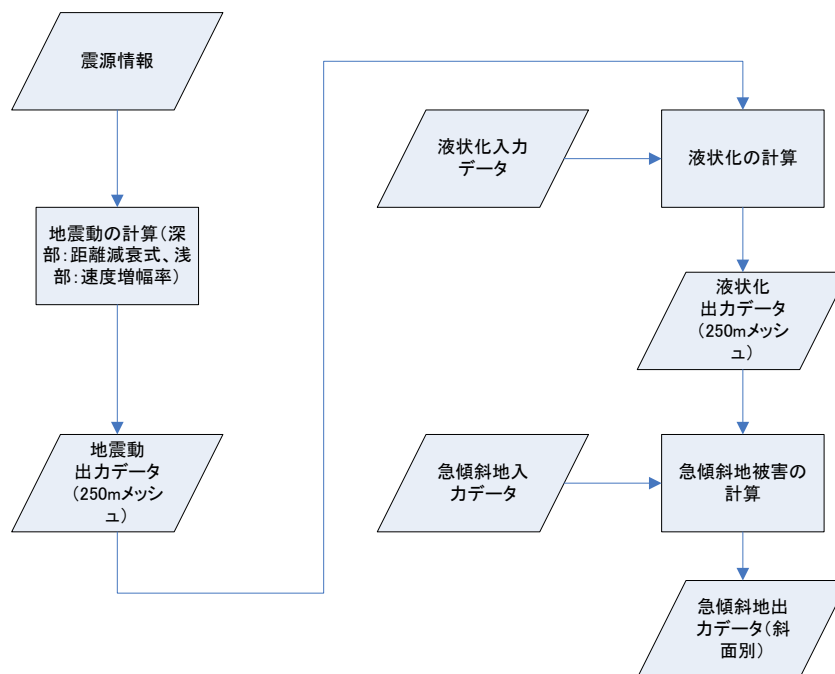
図 2.1.1-1 地震動・液状化・土砂災害被害予測フロー
