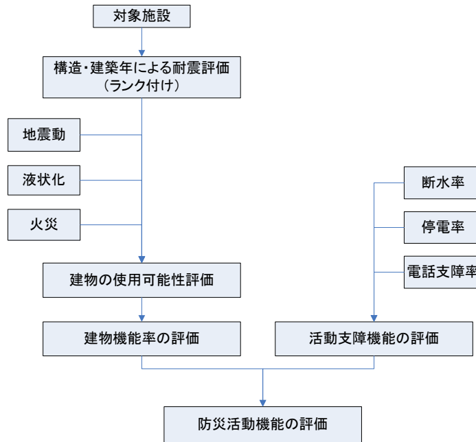
図 9.1-1 重要施設の評価フロー
