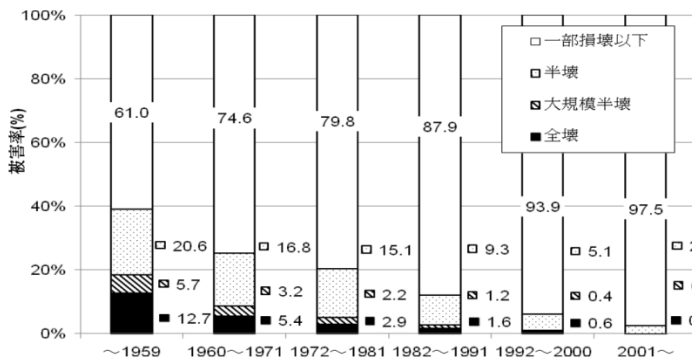
図 1.2.1-2 建築年代別の住宅被害率（木造）出典：長尾・山崎（2011）、『2007 年新潟県中越沖地震における柏崎市建物被害の空間分析』
