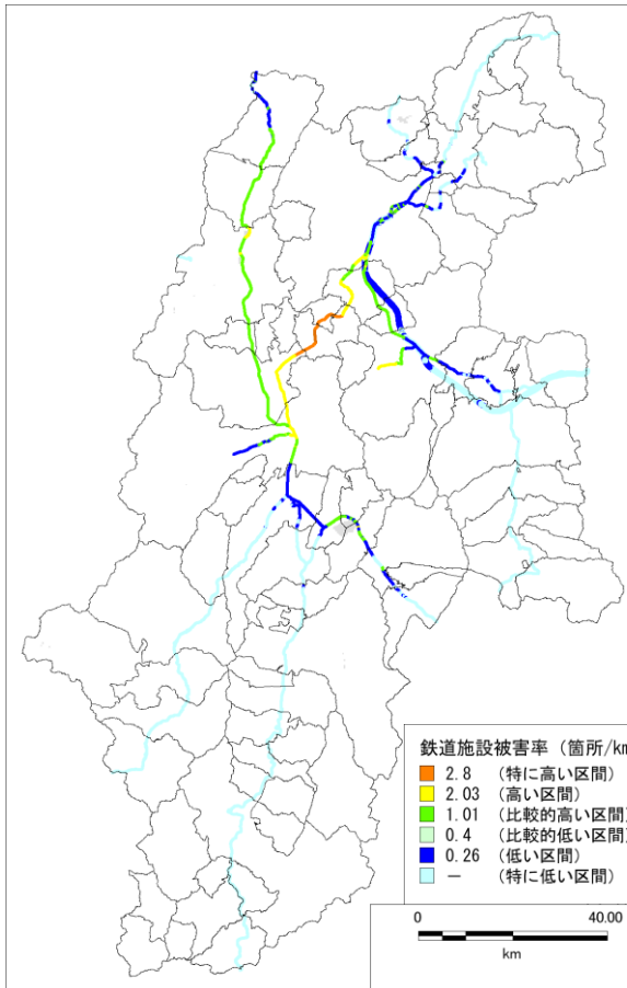
図 5.2-4 糸魚川-静岡構造線断層帯の地震(北側)における鉄道施設被害率分布図
