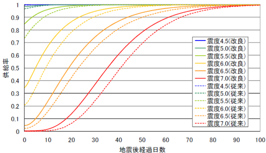
図 6.1-4 上水道の計測震度に対する供給率曲線の予測
