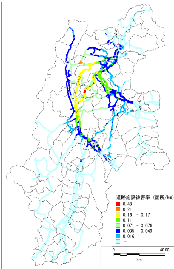
図 5.1-4 糸魚川-静岡構造線断層帯の地震(北側)における道路施設被害率分布図
