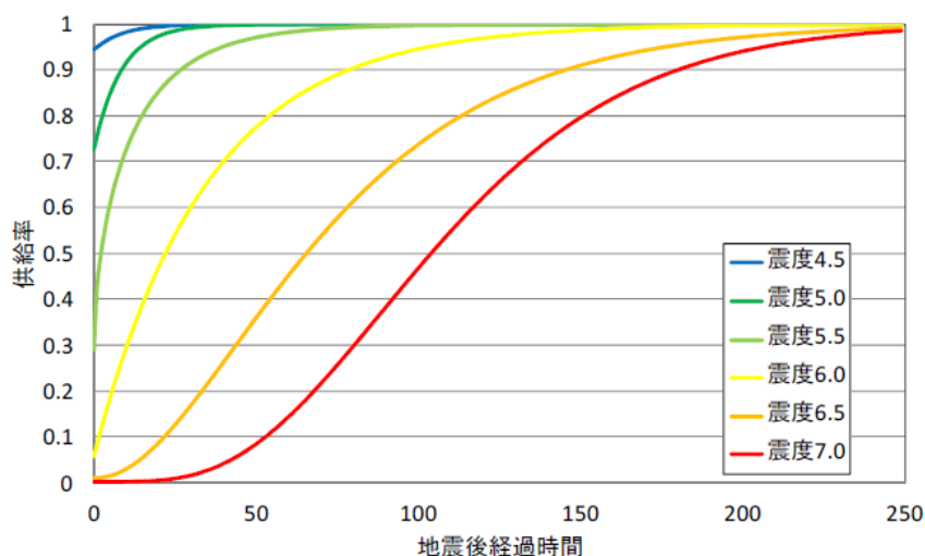
図 6.4-4 電力の計測震度に対する供給率曲線の予測
