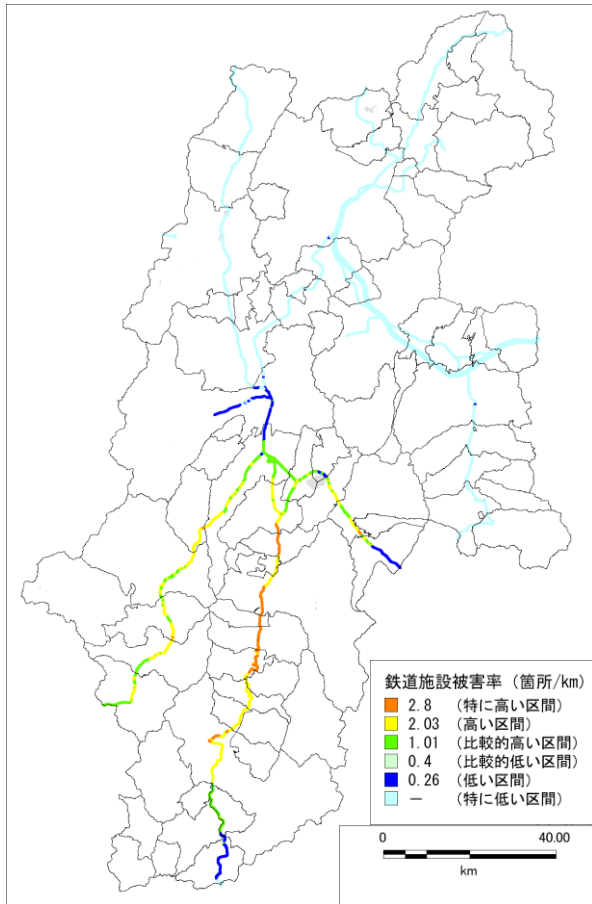
図 5.2-6 伊那谷断層帯(主部)の地震(ケース3)における鉄道施設被害率分布図
