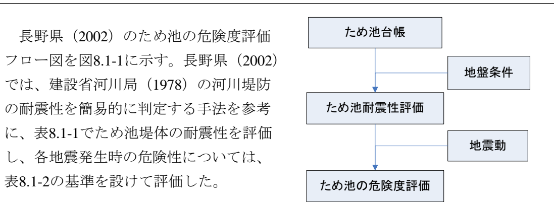
図8.1-1 ため池の危険度評価フロー （長野県，2002）
